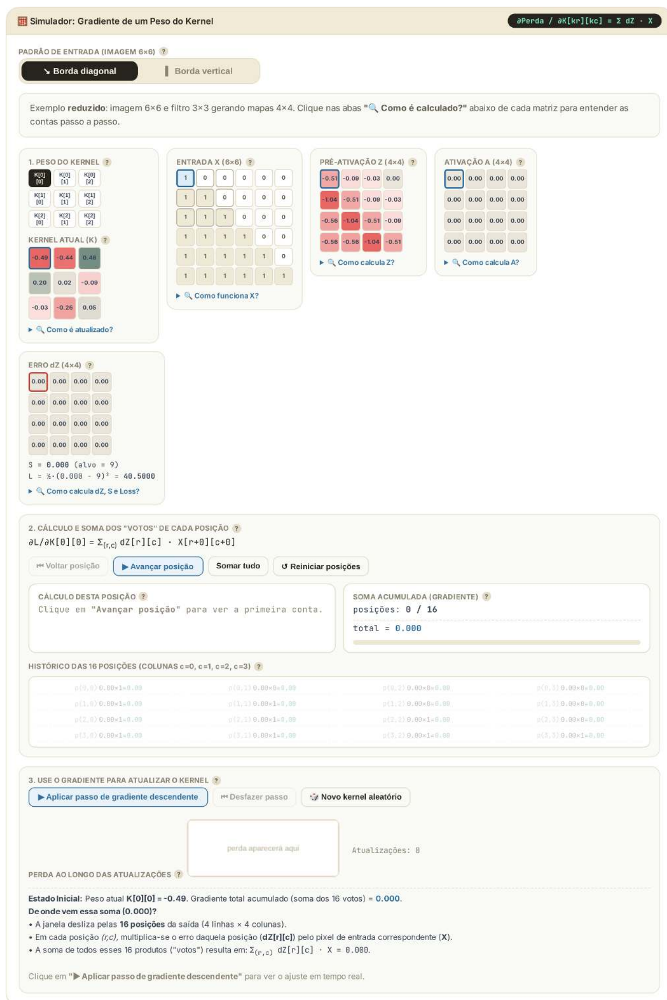
Figura 9.12: Simulador interativo do cálculo do gradiente de um peso do kernel convolucional com explicação detalhada da soma do gradiente inicial e alinhamento à esquerda.
