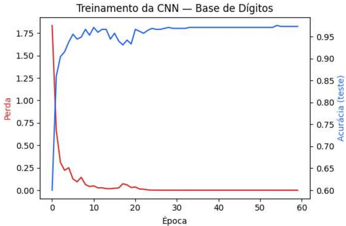
Figura 9.13: Curva de treinamento de uma CNN simples na base de dígitos: perda de treinamento e acurácia no conjunto de teste ao longo das épocas.
