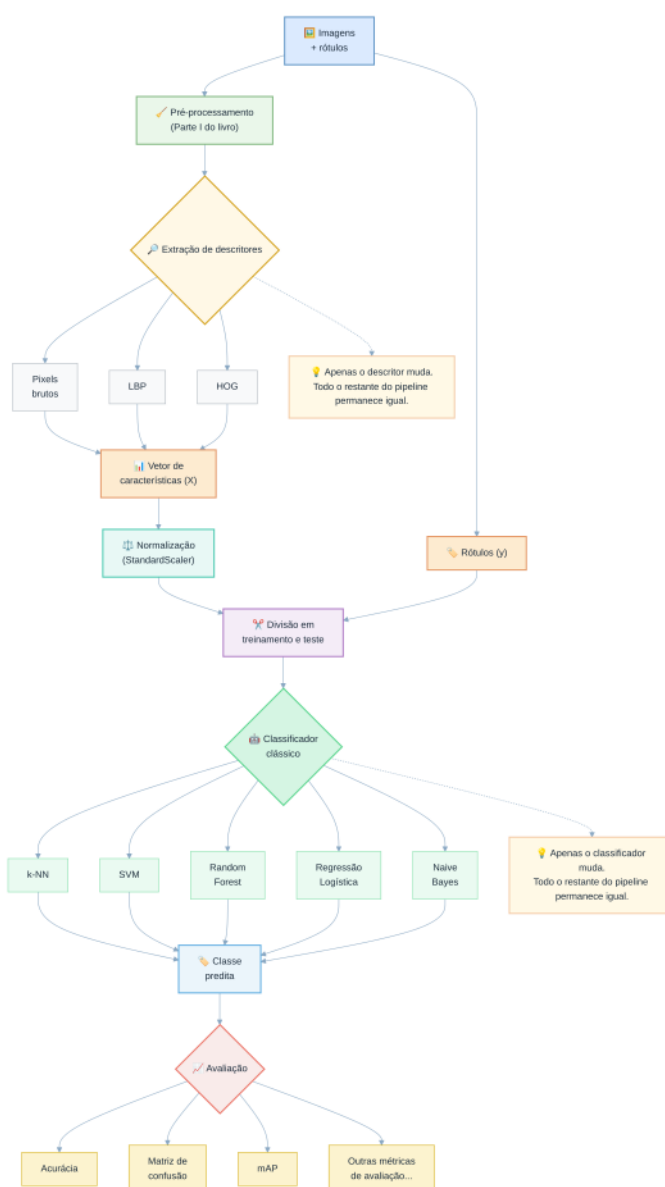
Figura 7.4: Mapa conceitual do processo de classificação de imagens utilizando descritores clássicos (LBP, HOG, pixels brutos) e classificadores tradicionais (k-NN, SVM, Random Forest, etc.). Não se aplica a modelos de deep learning (CNNs, YOLO), que aprendem features end-to-end diretamente dos pixels.
