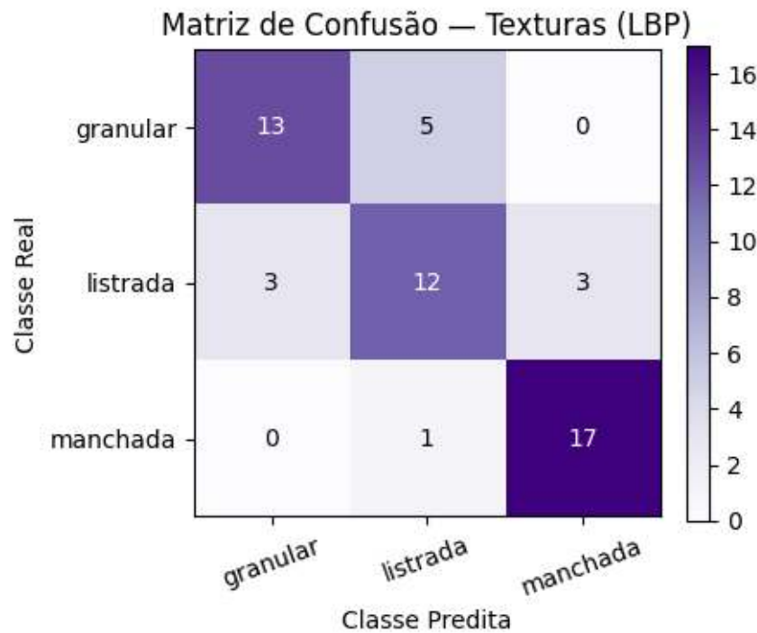
Figura 7.15: Matriz de confusão do classificador k-NN treinado com descritores LBP para as três classes de textura sintética, incluindo ruído e variabilidade intra-classe.
