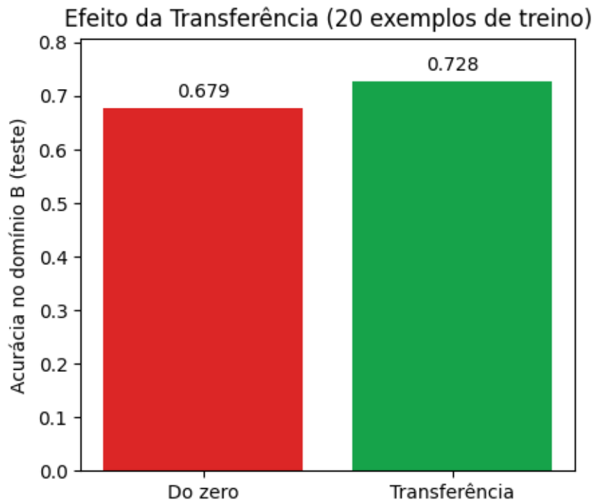
Figura 9.20: Comparação de acurácia entre treinar do zero e reaproveitar (transferir) um extrator de características já treinado, ambos com o mesmo pequeno número de exemplos rotulados na tarefa de destino.
