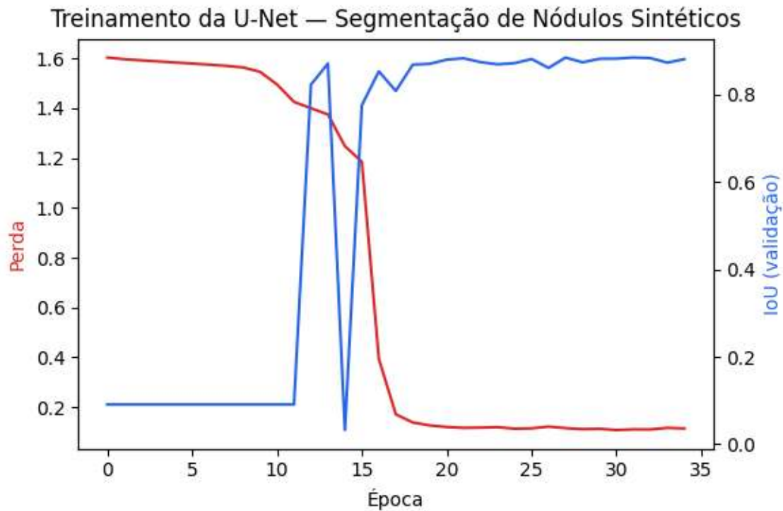
Figura 9.25: Curva de treinamento da U-Net compacta: perda de treinamento (entropia cruzada binária combinada à perda Dice) e IoU médio no conjunto de validação ao longo das épocas.
