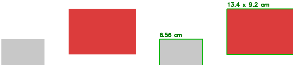
Figura 9.28: Medição de um objeto a partir de uma referência de escala conhecida (um cartão de 8,56 cm de largura).
