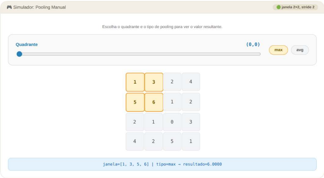
Figura 9.31: Simulador: Pooling Manual (máximo vs. média)
