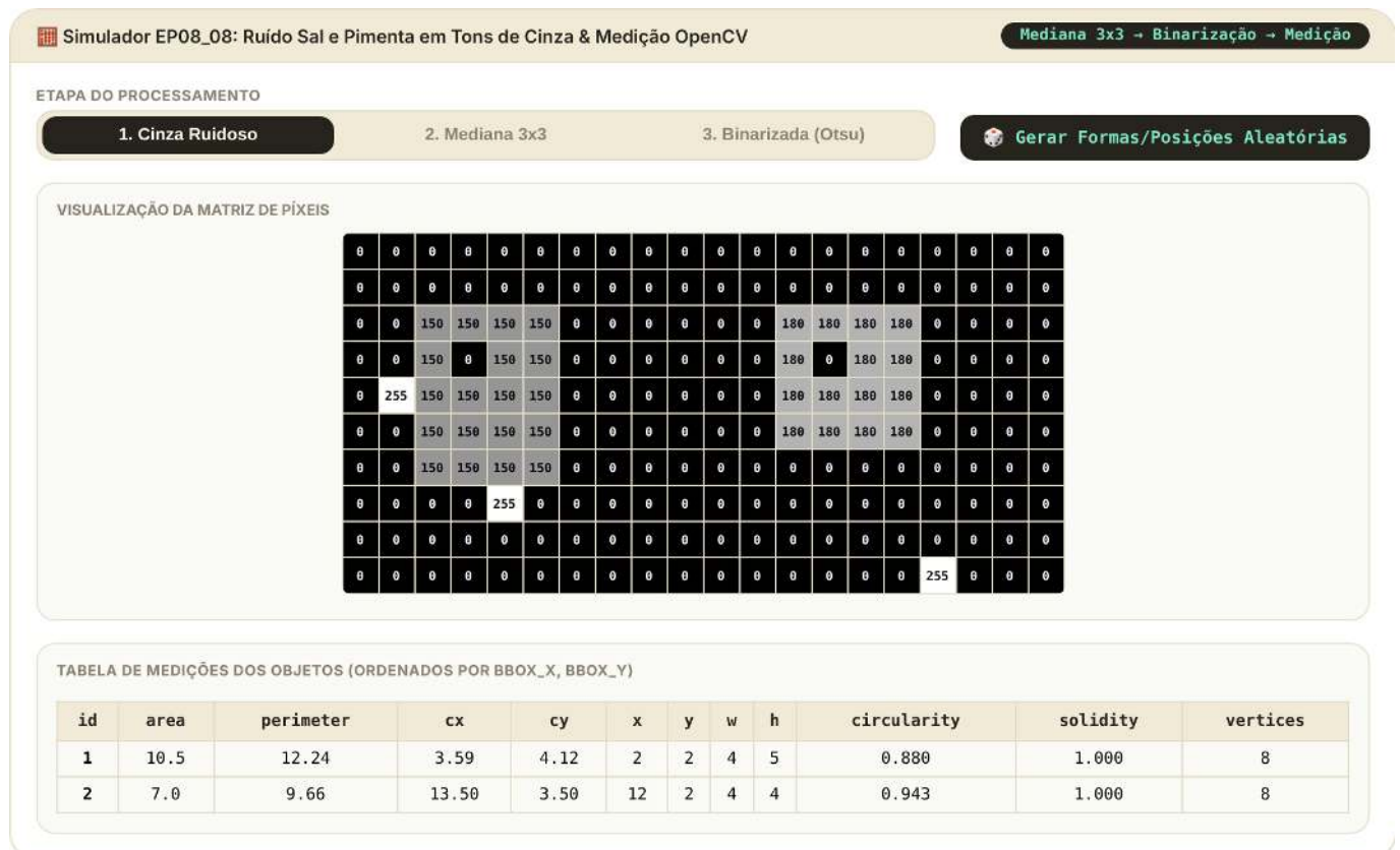
Figura 8.22: Simulador EP08_08: Filtragem de Mediana em Tons de Cinza e Medição de Objetos OpenCV
