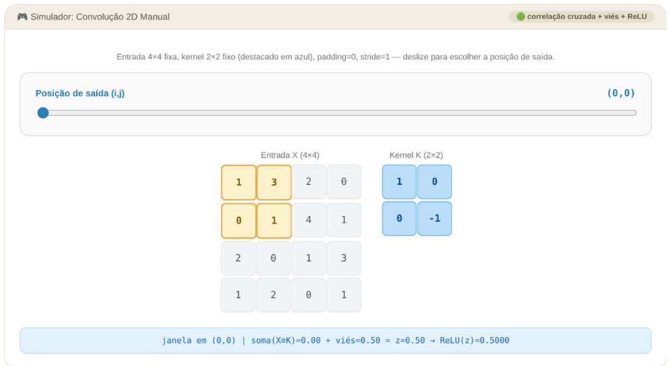
Figura 9.41: Simulador EP09_01: Convolução 2D Manual (correlação cruzada + viés + ReLU)
