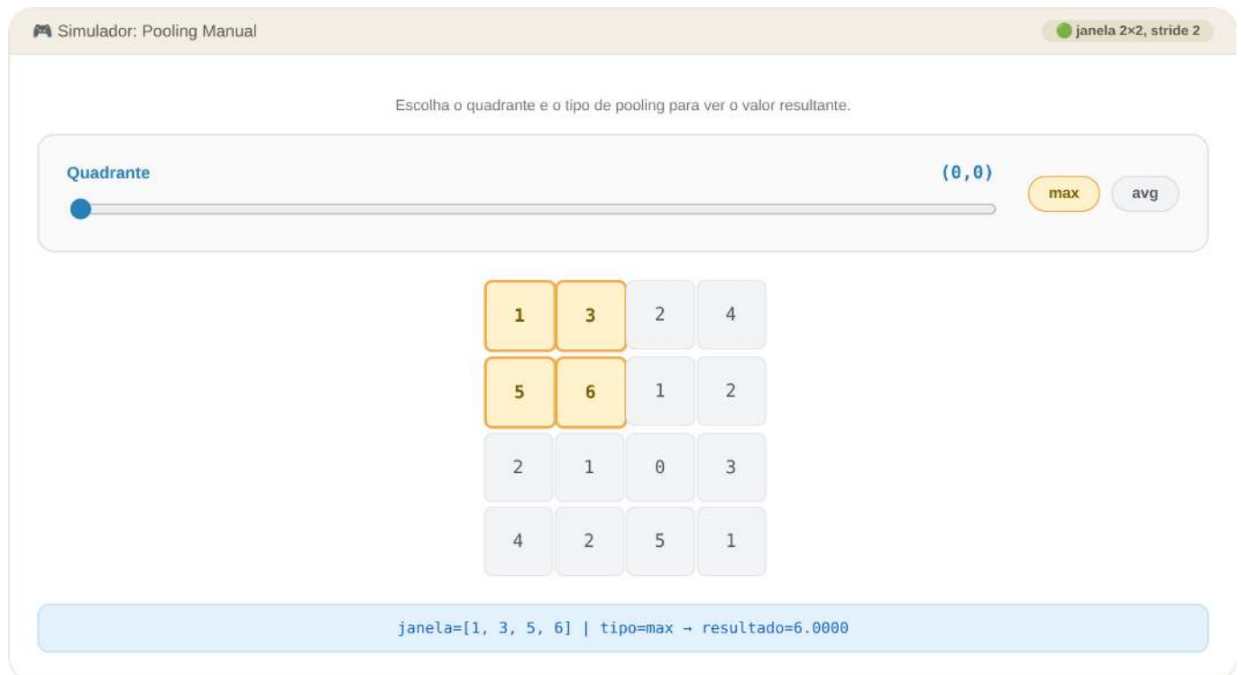
Figura 9.42: Simulador EP09_02: Pooling Manual (máximo vs. média)
