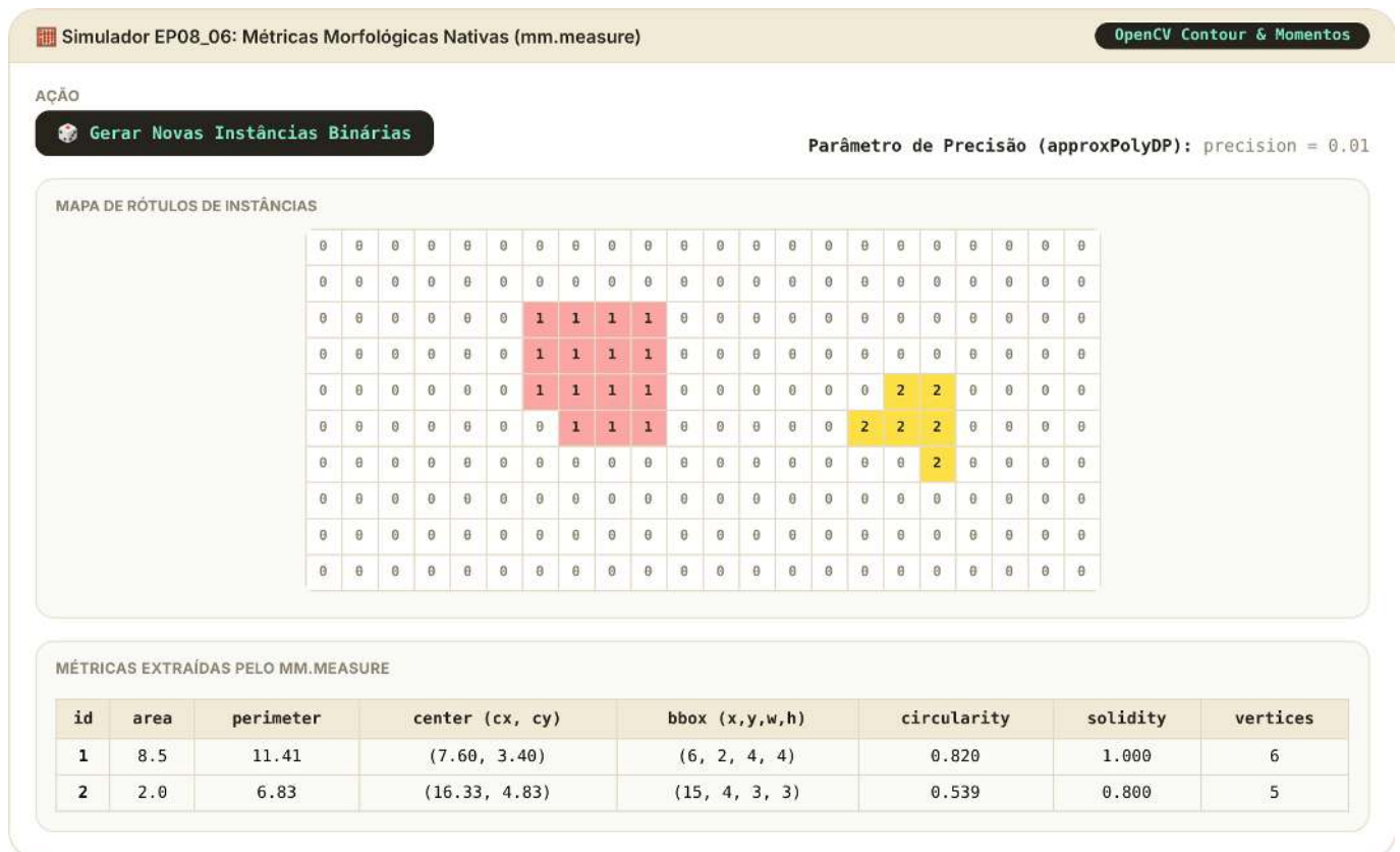
Figura 8.20: Simulador EP08_06: Extração de Bounding Boxes, Centroides e Propriedades com mm.measure
