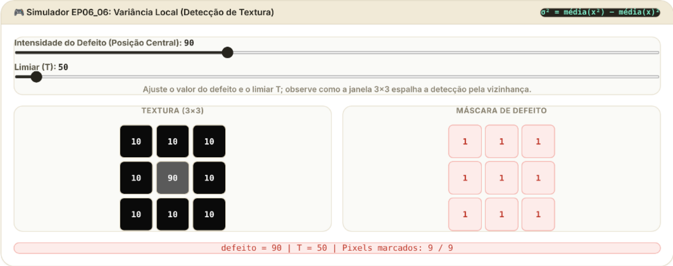
Figura 6.26: Simulador EP06_06: Mapa de Variância Local para Detecção de Textura
