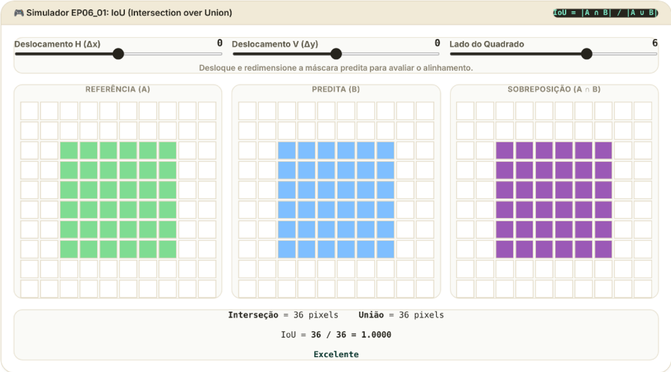
Figura 6.21: Simulador EP06_01: IoU entre máscara de referência e máscara predita
