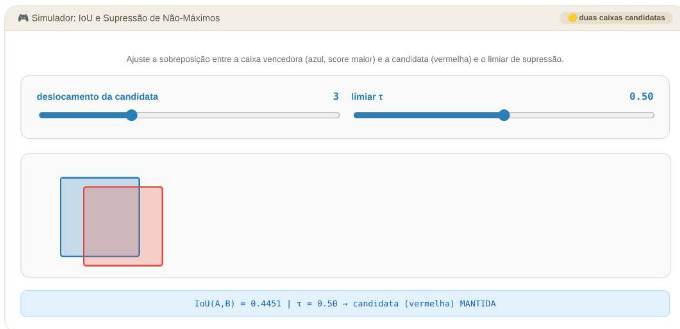
Figura 9.13: Simulador: IoU e Supressão de Não-Máximos
