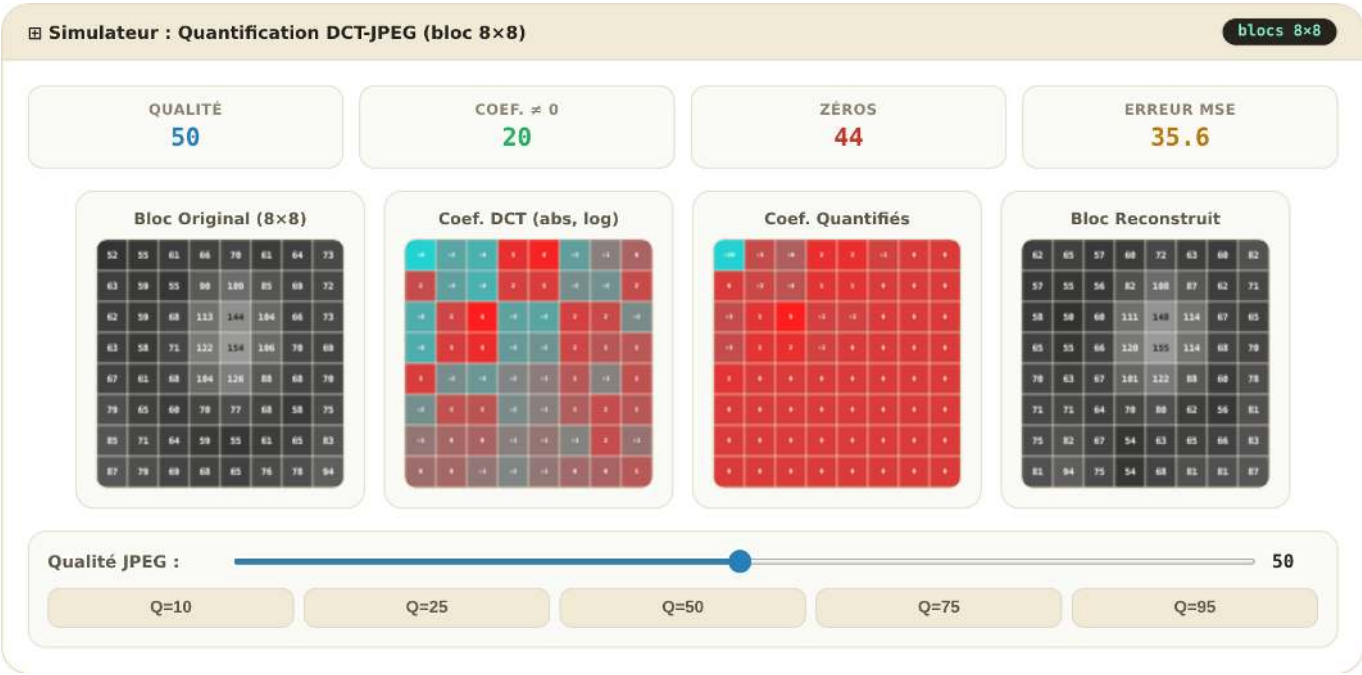
Figure 5.26: Simulateur interactif de compression DCT-JPEG : ajustez le facteur de qualité et visualisez en temps réel les coefficients nuls, le bloc reconstruit et l’erreur de quantification.
