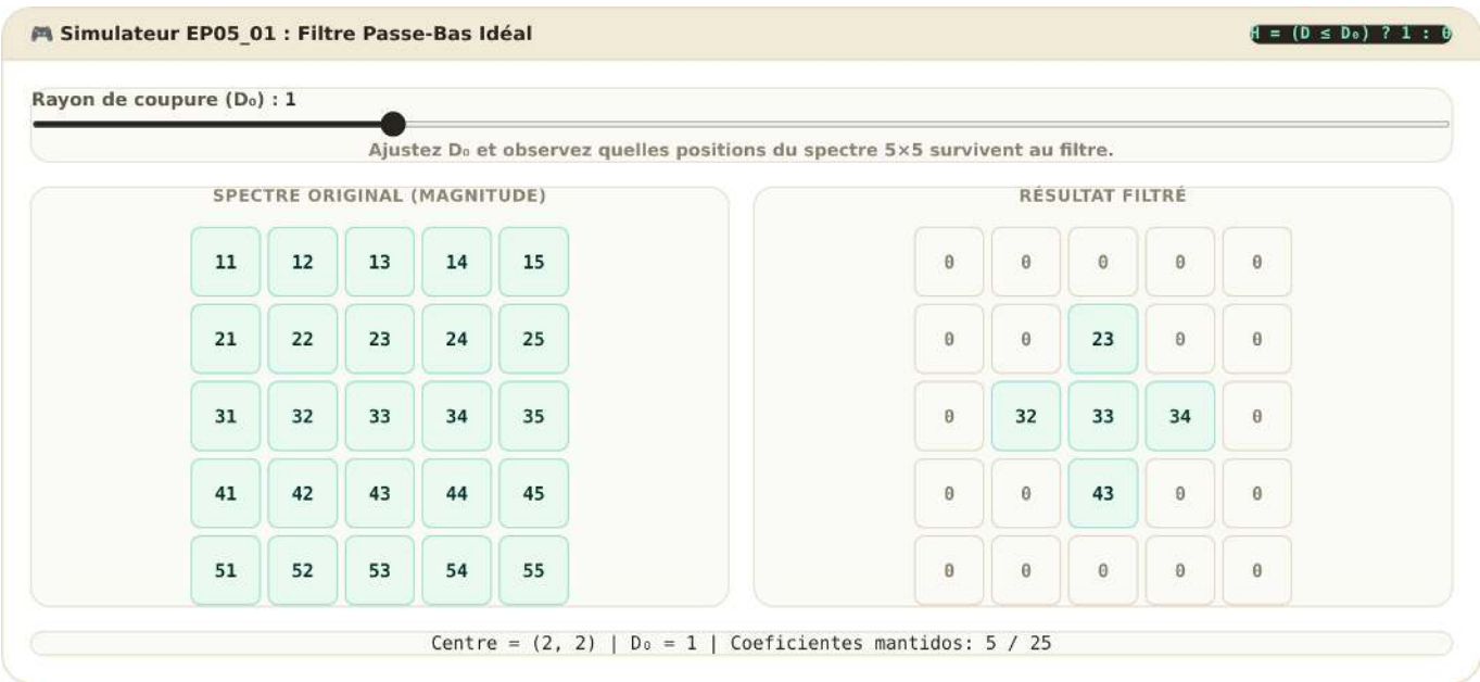
Figure 5.32: Simulateur EP05_01 : Filtre passe-bas idéal dans le spectre
