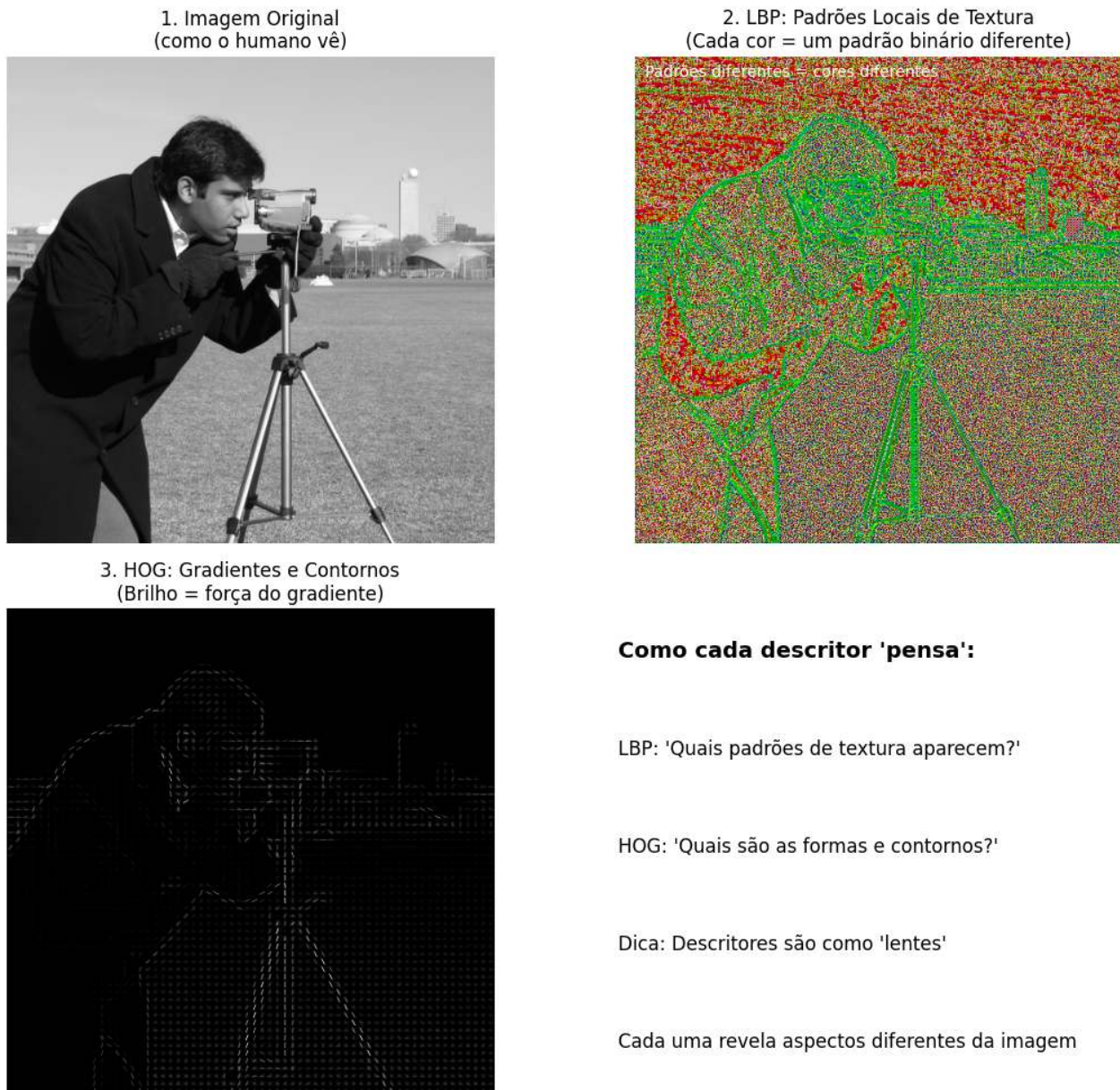
Figura 7.2: Comparação visual de diferentes descritores aplicados à mesma imagem. Cada descritor revela aspectos distintos da cena.
