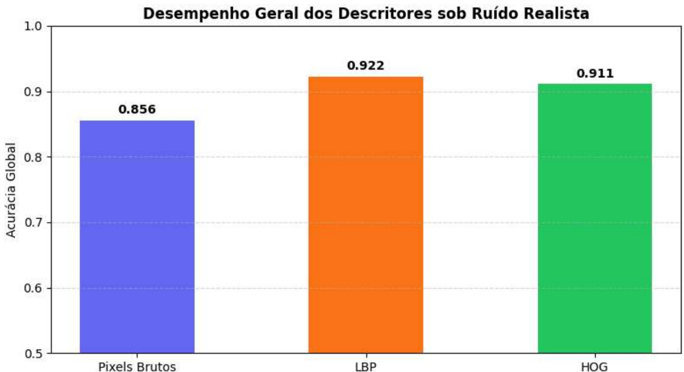
Figura 7.5: Comparação detalhada de acurácia global em cenário realista. Observe como os descritores extraídos estruturalmente (LBP e HOG) superam o uso de intensidades puras de pixels brutos.
