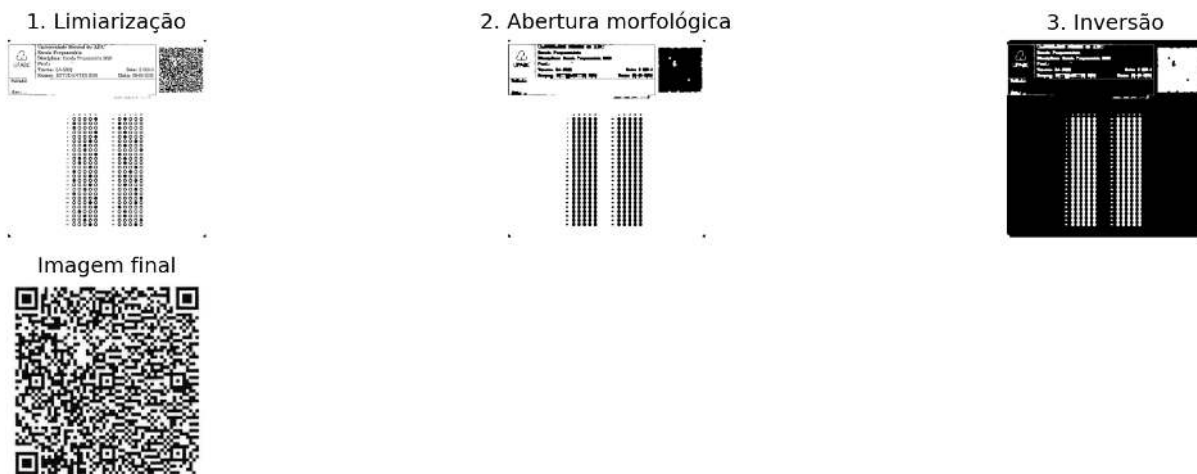
Figura 6.10: Pipeline de processamento do QRCode : limiarização, abertura morfológica, inversão e recorte final para decodificação.
