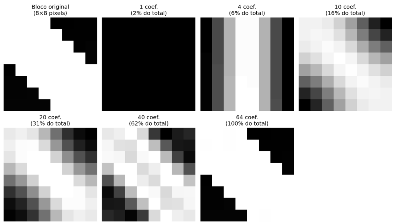
Figura 5.24: DCT 2D em bloco 8x8: coeficientes e reconstrução progressiva.
