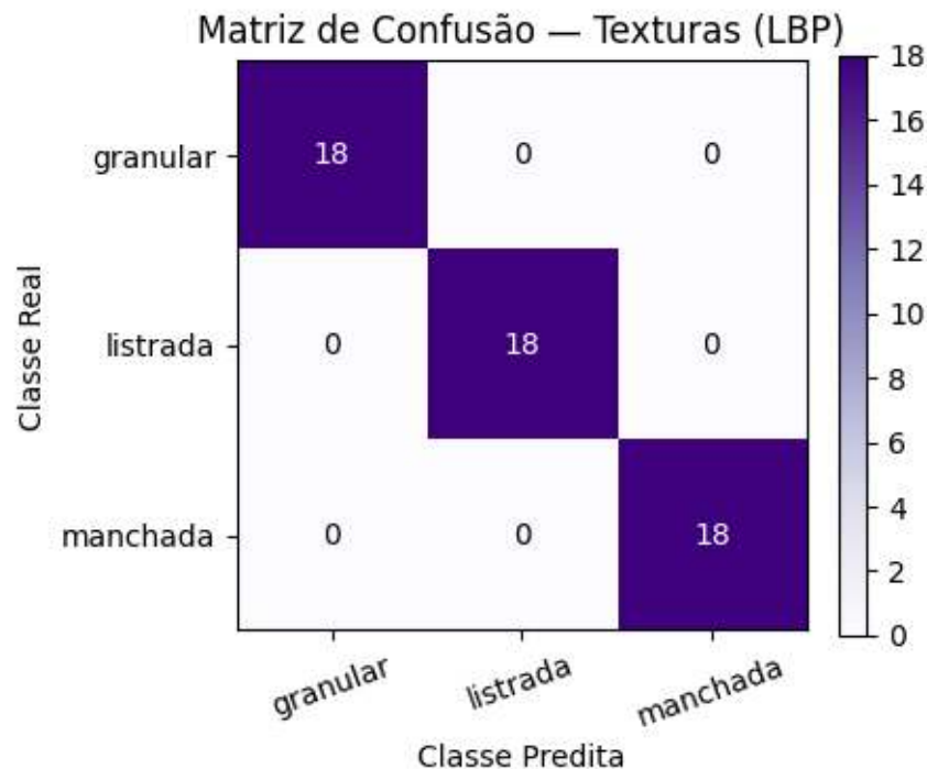
Figura 7.15: Matriz de confusão do classificador k-NN treinado com descritores LBP para as três classes de textura sintética.
