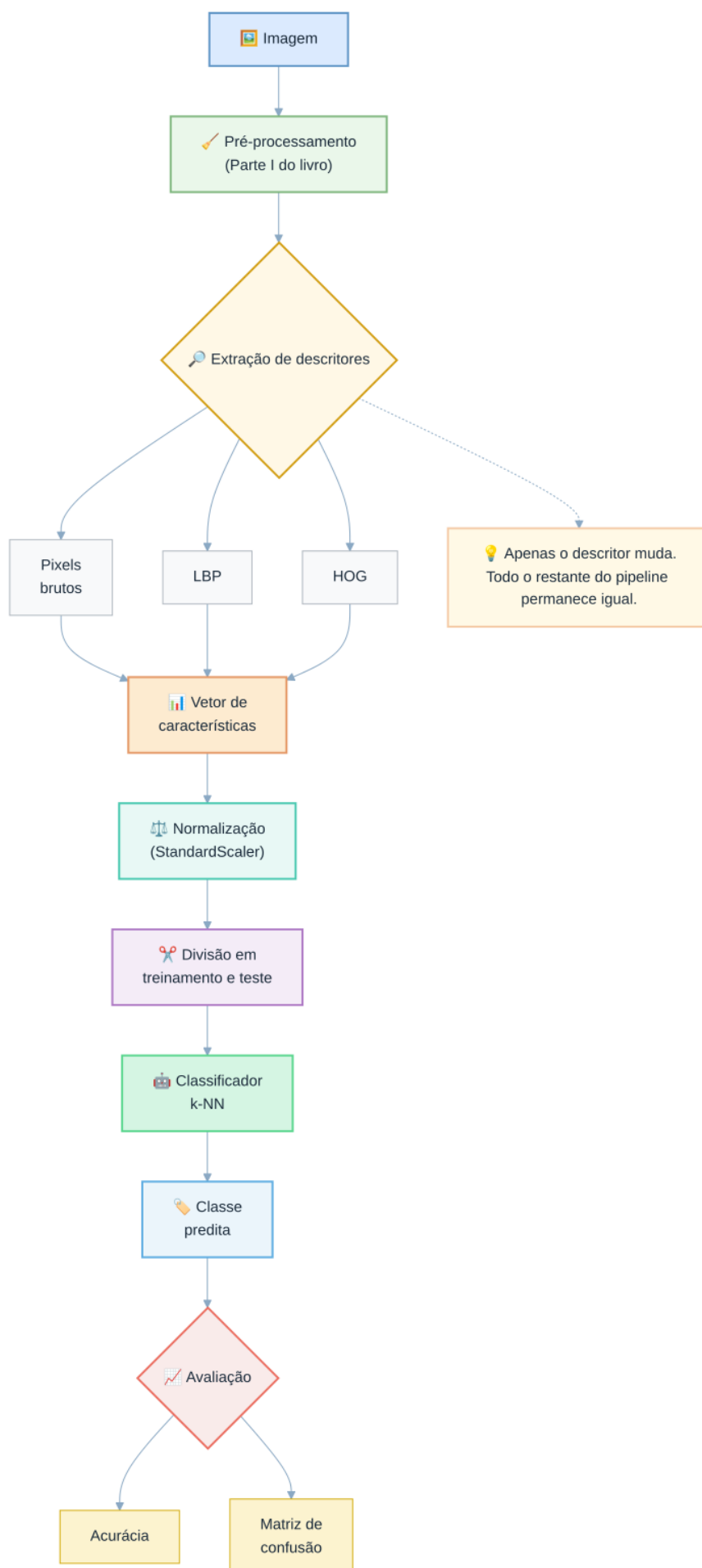
— Figura 7.4: Mapa conceitual do processo de classificação de imagens utilizando descritores clássicos. —
