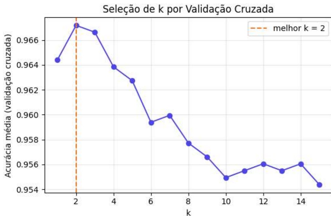
Figura 7.12: Acurácia média por validação cruzada (5 partições) em função do parâmetro k , para a base de dígitos com vetores de intensidade brutos.
