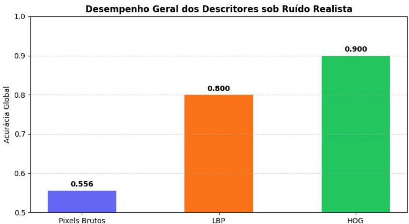
Figura 7.6: Comparação detalhada de acurácia global em cenário realista. Observe como os descritores extraídos estruturalmente (LBP e HOG) superam o uso de intensidades puras de pixels brutos.
