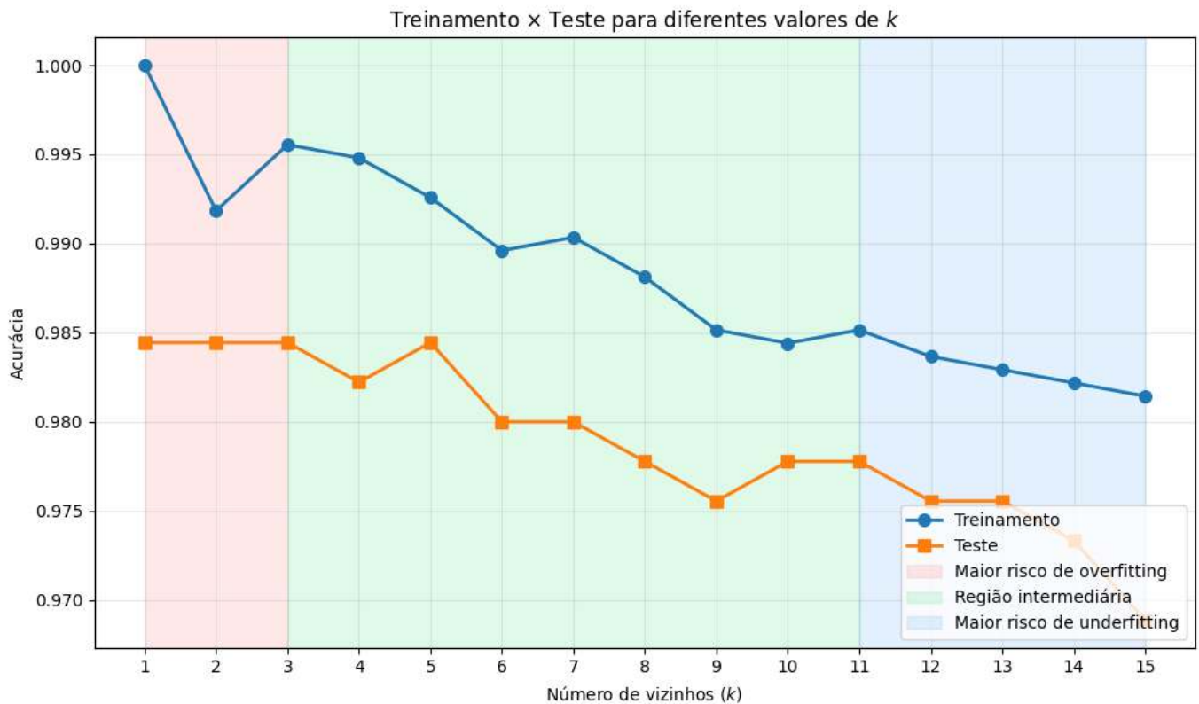
Figura 7.13: Acurácia nos conjuntos de treinamento e teste para diferentes valores de k . As regiões coloridas representam, de forma conceitual, a tendência de comportamento do classificador: maior risco de sobreajuste (vermelho), região intermediária (verde) e maior risco de subajuste (azul).
