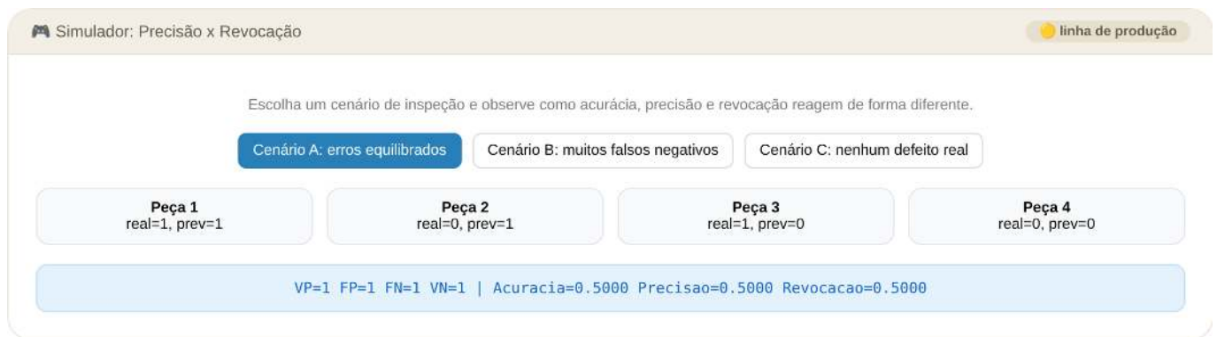
Figura 7.20: Simulador: Precisão x Revocação
