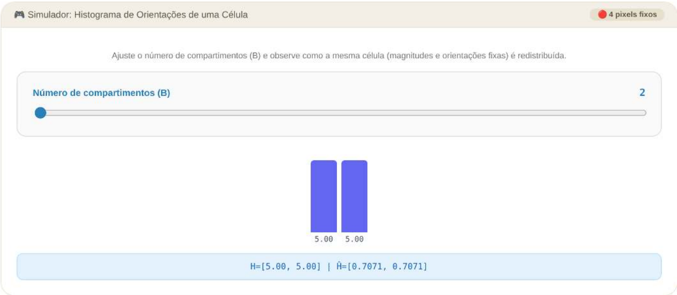
Figura 7.22: Simulador: Histograma HOG de uma Celula
