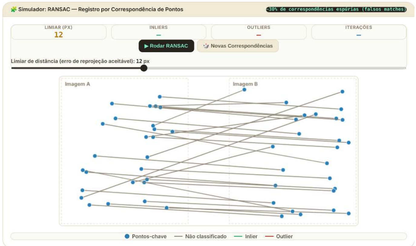
Figura 8.7: Simulador interativo do RANSAC aplicado ao registro de imagens: pontos-chave de duas imagens são casados por um descritor, algumas correspondências são espúrias ( outliers ), e o RANSAC estima a transformação de similaridade que alinha a maioria delas.
