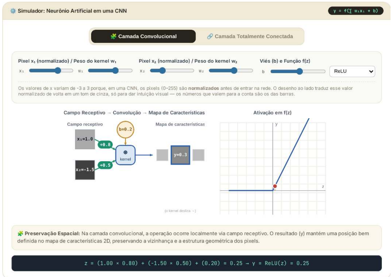
Figura 9.3: Simulador interativo do Neurônio Artificial em contexto de CNN: alterne entre um neurônio de camada convolutacional (onde x_i são intensidades de pixel em um campo receptivo e w_i são pesos do kernel ) e um neurônio de camada totalmente conectada, ajustando entradas, pesos, viés e função de ativação para visualizar o cálculo de z e da saída y em tempo real.
