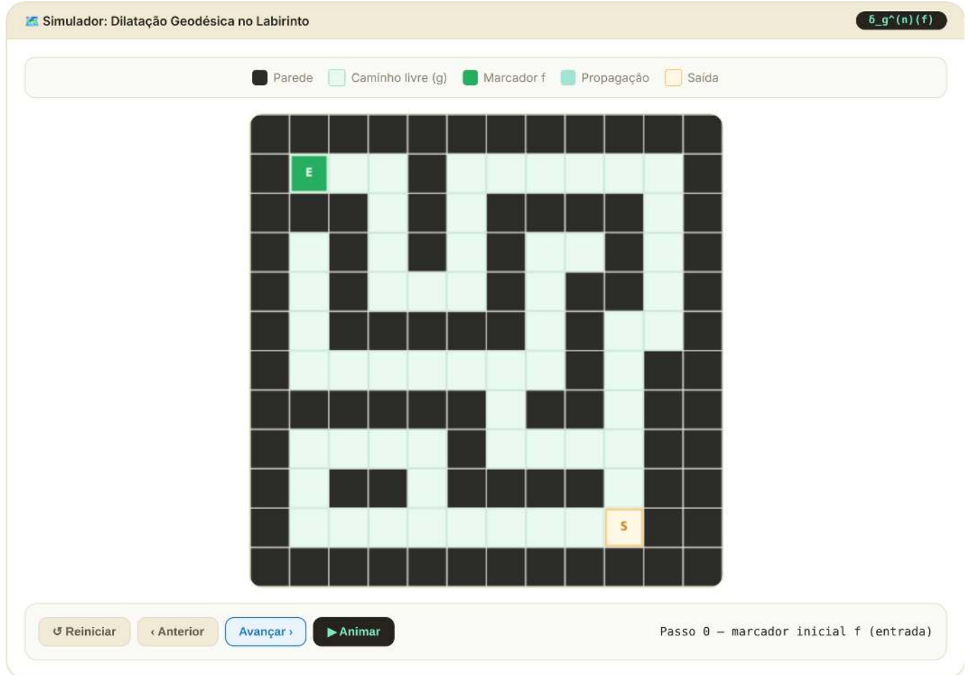
Figura 4.7: Simulador interativo de dilatação geodésica: o marcador f (verde) propaga-se passo a passo pelos caminhos livres da máscara g , sem atravessar paredes — ilustrando como \hat{g}^{(n)}(f) encontra a saída do labirinto.
