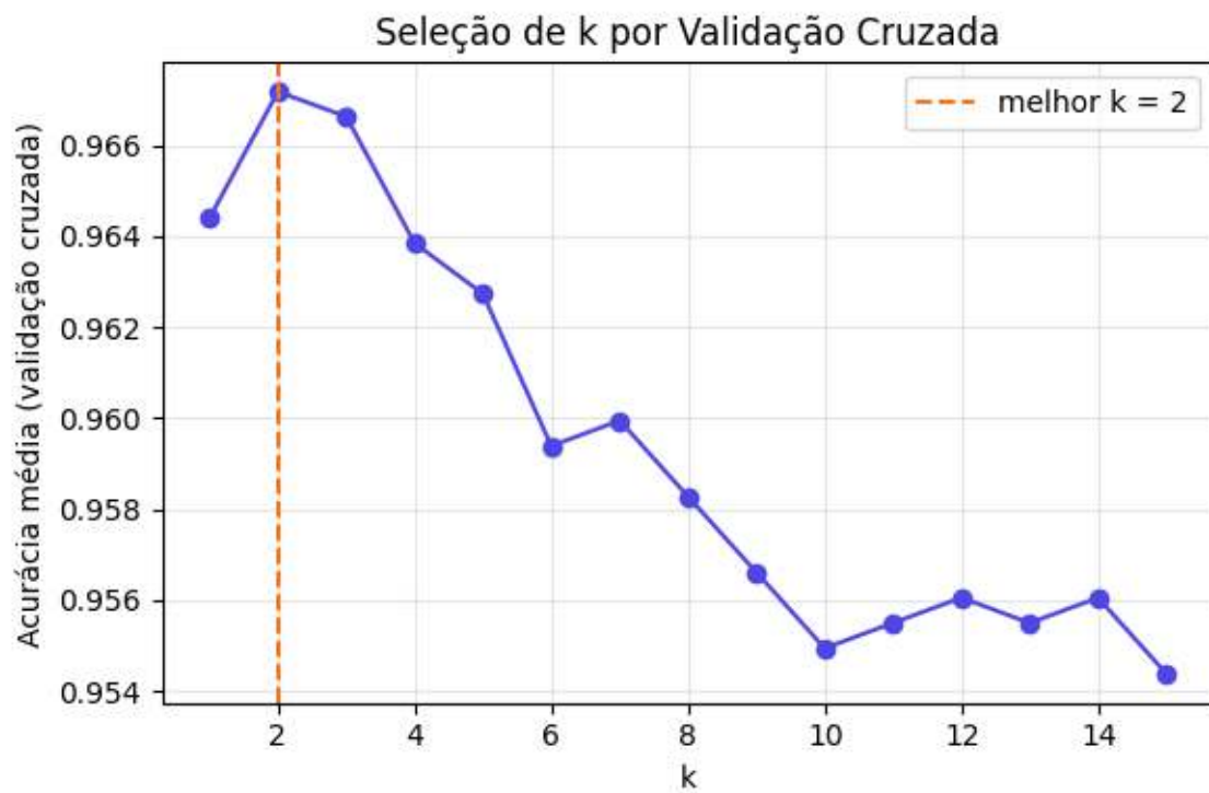
Figura 7.14: Acurácia média por validação cruzada (5 partições) em função do parâmetro k , para a base de dígitos com vetores de intensidade brutos.
