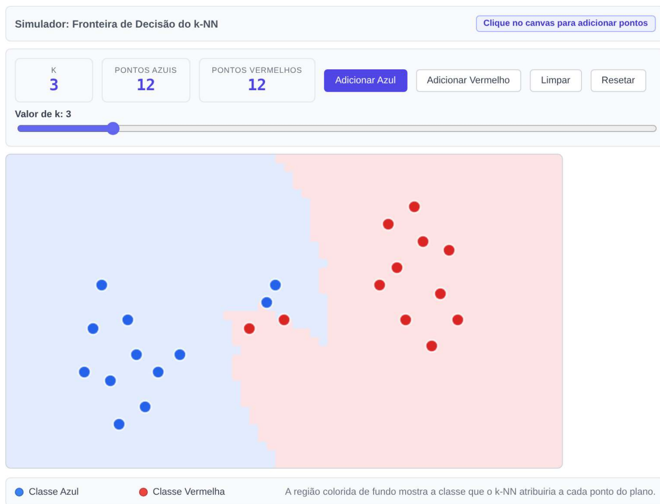
Figura 7.10: Simulador interativo da fronteira de decisão do k-NN: adicione pontos de treinamento e ajuste o valor de k para observar o efeito sobre a região de decisão.
