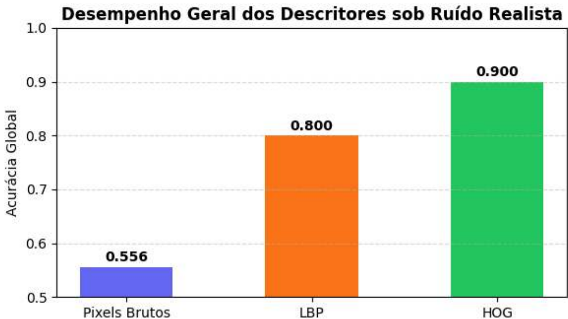
Figura 7.7: Comparação detalhada de acurácia global em cenário realista. Observe como os descritores extraídos estruturalmente (LBP e HOG) superam o uso de intensidades puras de pixels brutos.
