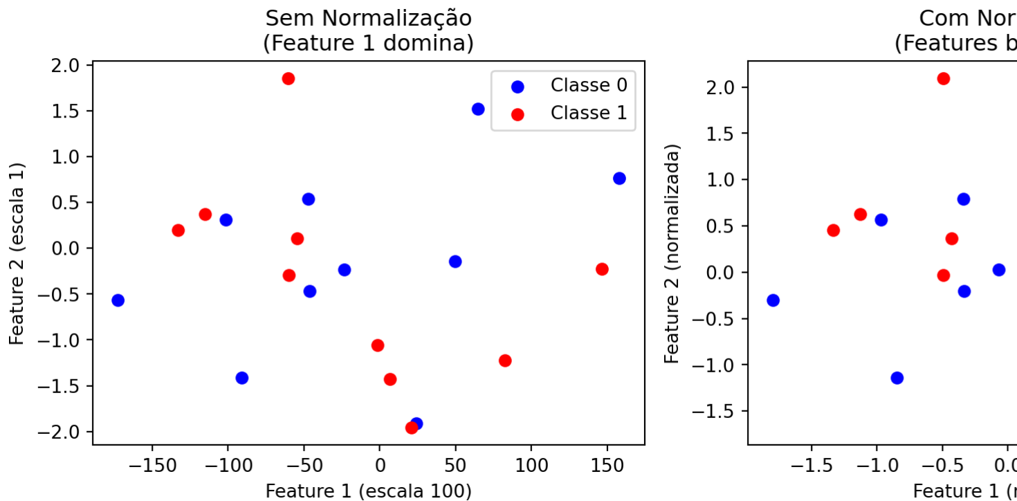
Figura 7.3: Importância da normalização de features para o classificador k-NN
