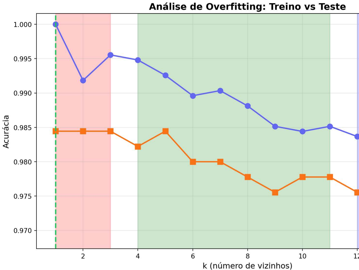
Figura 7.12: Análise de overfitting: comparação da acurácia entre treino e teste para diferentes valores de k
