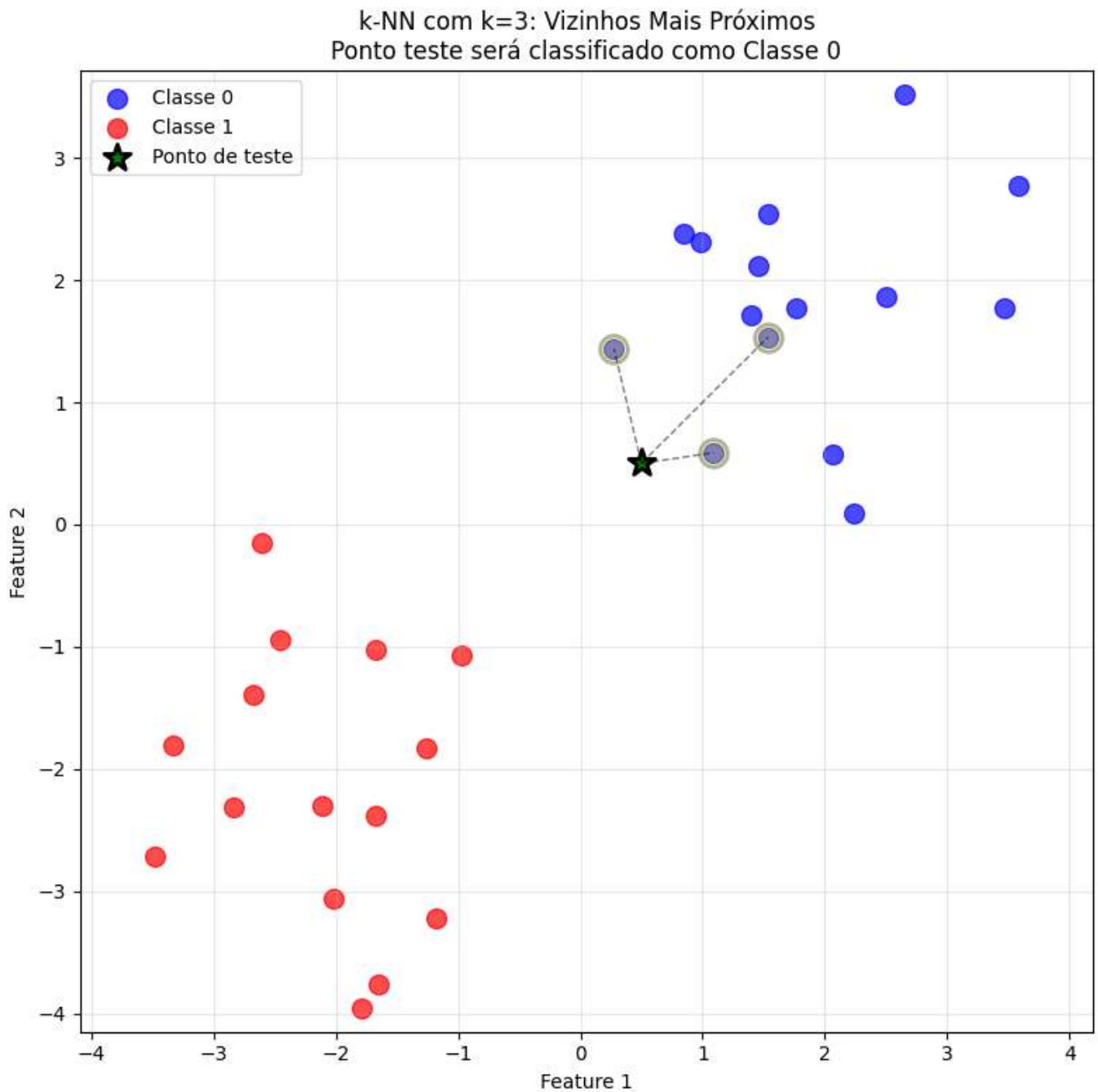
Figura 7.7: Visualização passo-a-passo da classificação k-NN, mostrando como os vizinhos mais próximos são identificados e como a votação decide a classe final.
