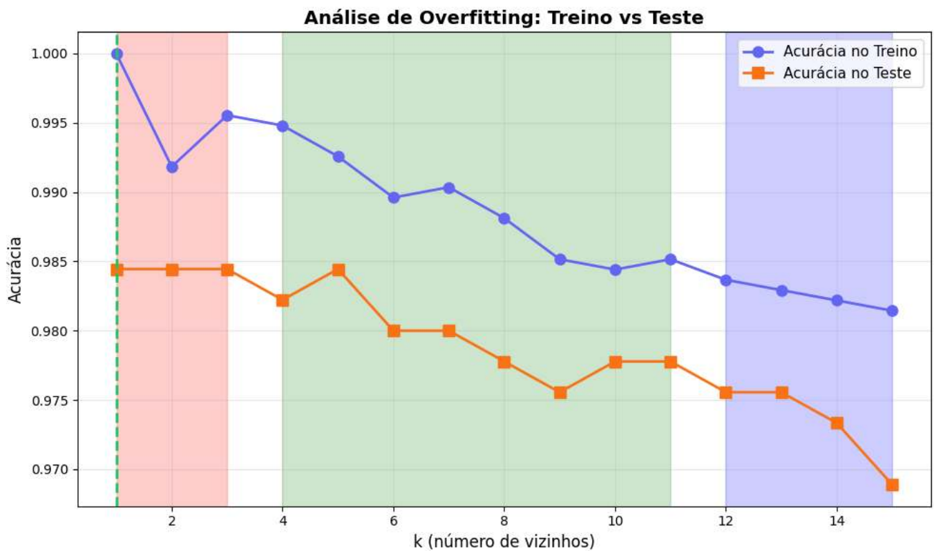
Figura 7.13: Análise de overfitting: comparação da acurácia entre treino e teste para diferentes valores de k
