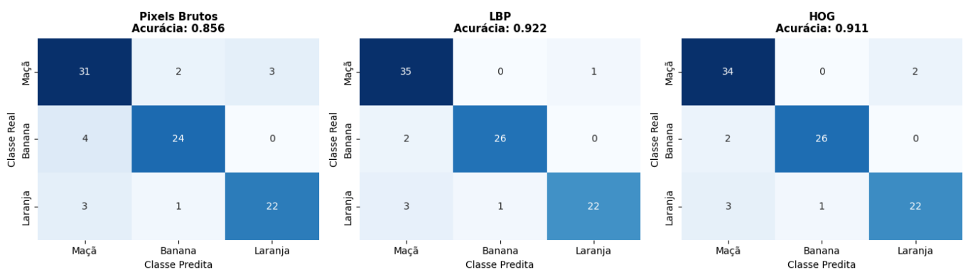
Figura 7.5: Matrizes de confusão obtidas pelo classificador k-NN utilizando três descritores diferentes. As linhas representam a classe real (Maçã, Banana e Laranja) e as colunas a classe predita. Quanto maior a concentração de valores na diagonal principal, melhor o desempenho do descritor.
