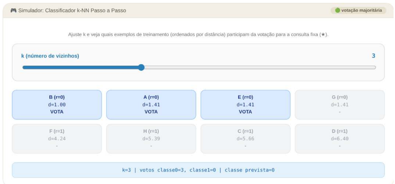
Figura 7.18: Simulador: Classificador k-NN Passo a Passo
