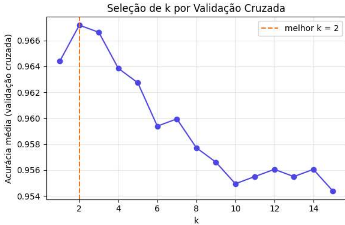
Figura 7.13: Acurácia média por validação cruzada (5 partições) em função do parâmetro k , para a base de dígitos com vetores de intensidade brutos.
