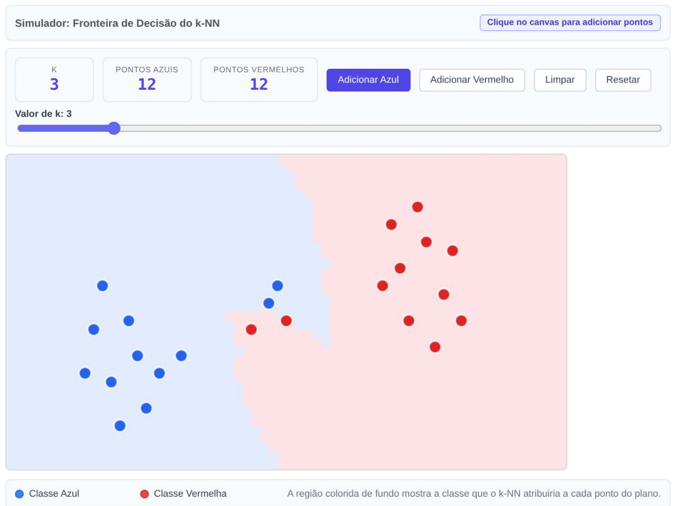
Figura 7.9: Simulador interativo da fronteira de decisão do k-NN: adicione pontos de treinamento e ajuste o valor de k para observar o efeito sobre a região de decisão.
