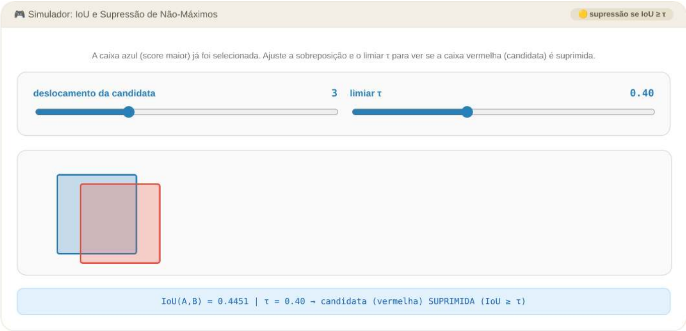
Figura 8.11: Simulador: IoU e Supressão de Não-Máximos
