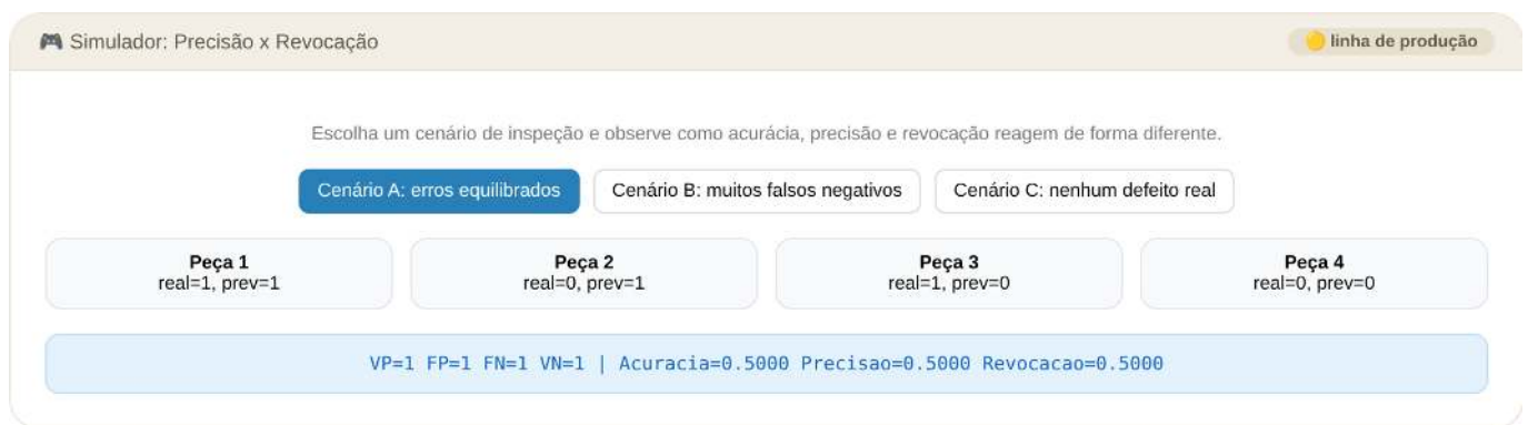
Figura 7.19: Simulador: Precisão x Revocação
