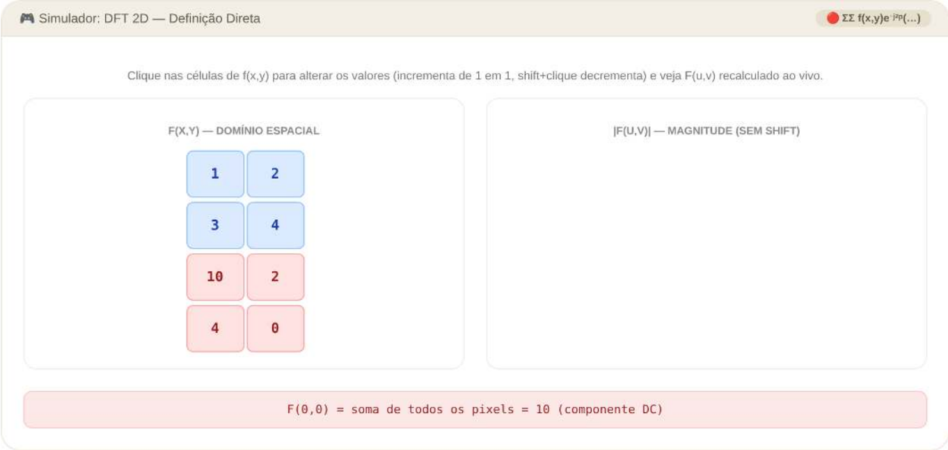
Figura 5.35: Simulador: DFT 2D manual
