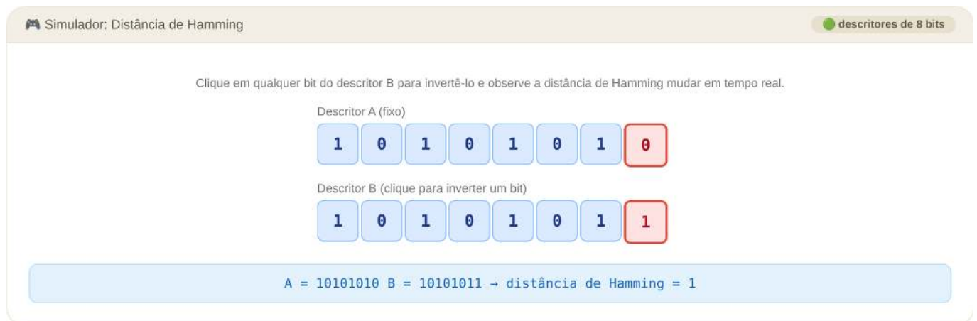
Figura 8.8: Simulador: Distância de Hamming entre Dois Descritores Binários
