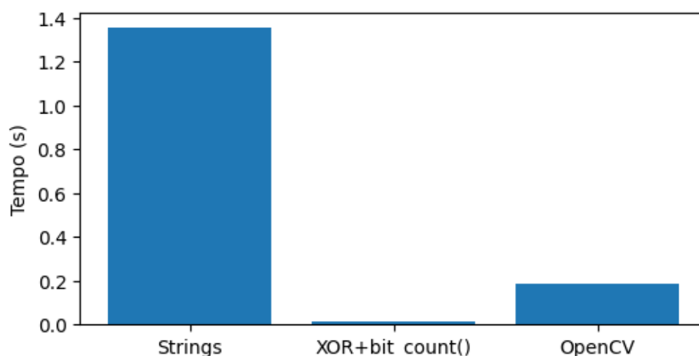
Figura 8.1: Comparação do desempenho de diferentes implementações da distância de Hamming.
