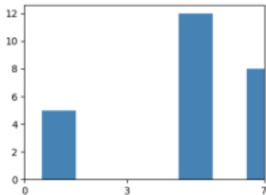
Histograma — Ecualizada
