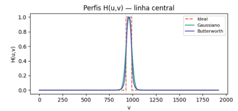
Perfis H(u,v)
