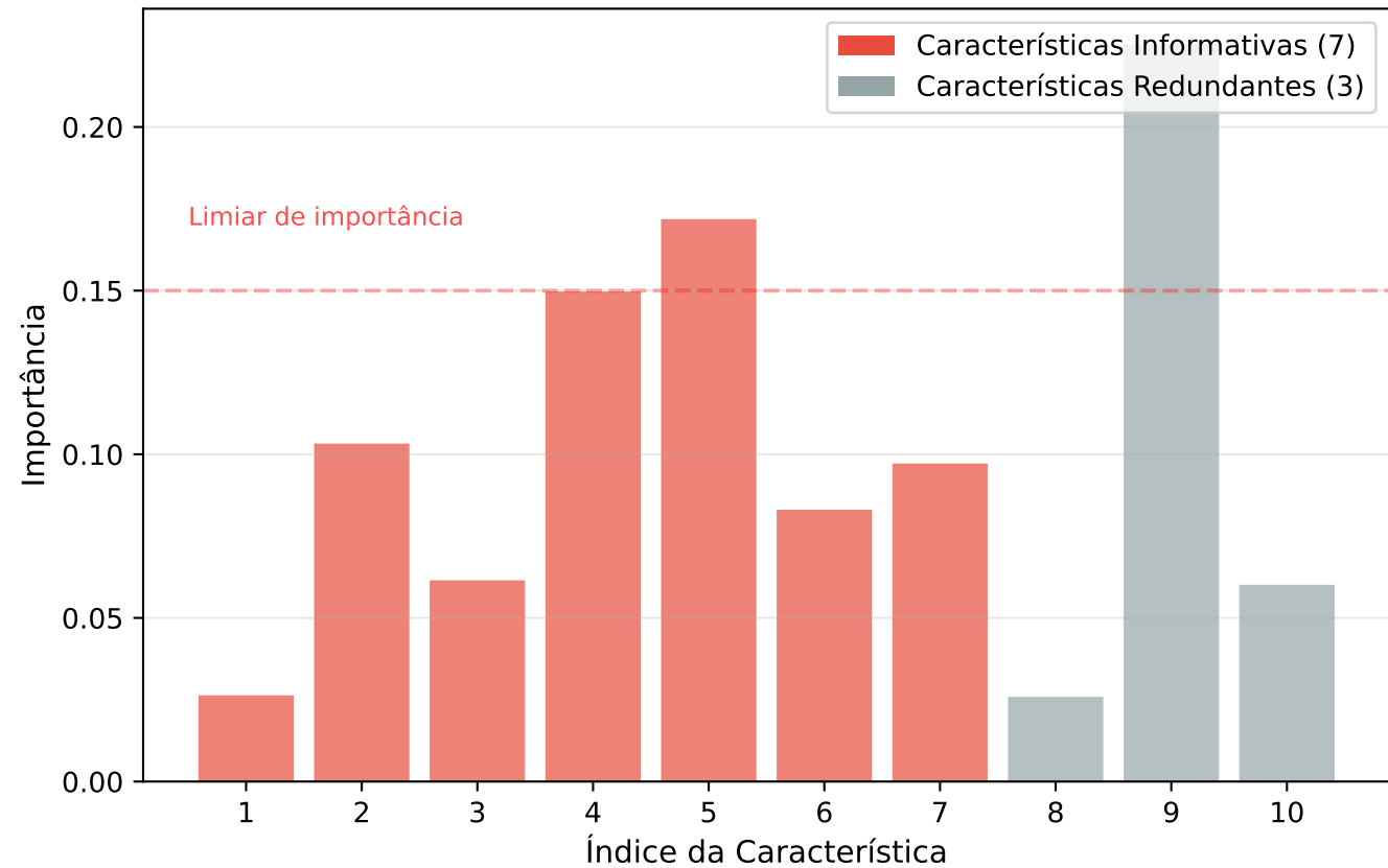
Importância de cada Característica para a Classificação
