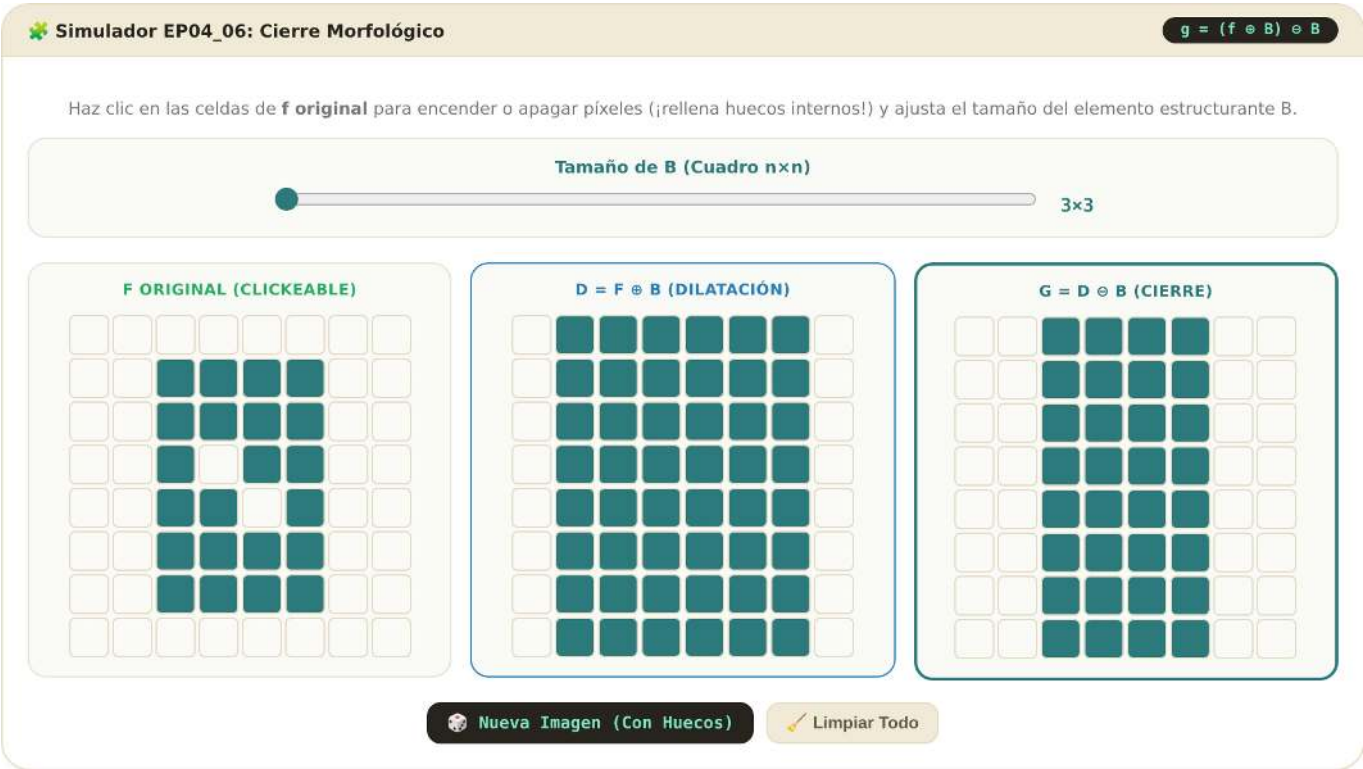
Figura 4.35: Simulador EP04_06: Cierre Morfológico ( g = (f \oplus B) \ominus B )
