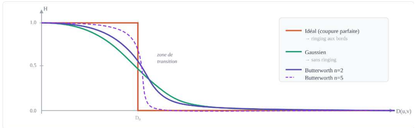
Figure 5.11: Filtros passe-bas.
