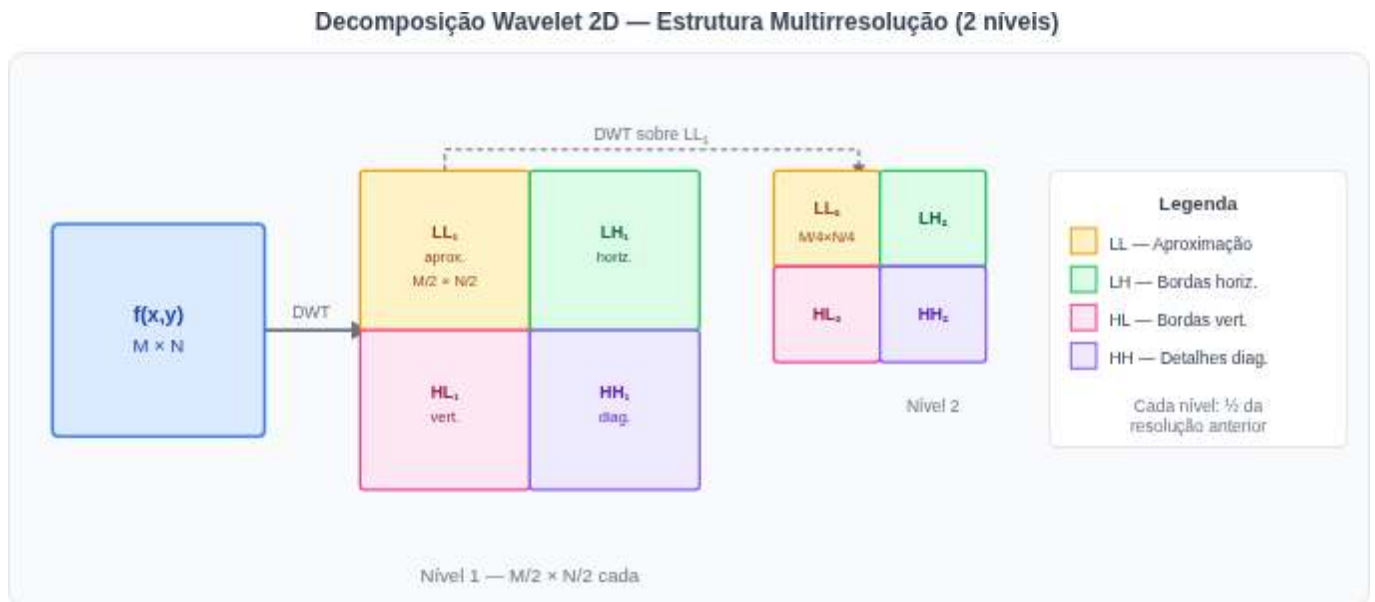
Figura 5.18: Diagrama da decomposição wavelet 2D em dois níveis.
