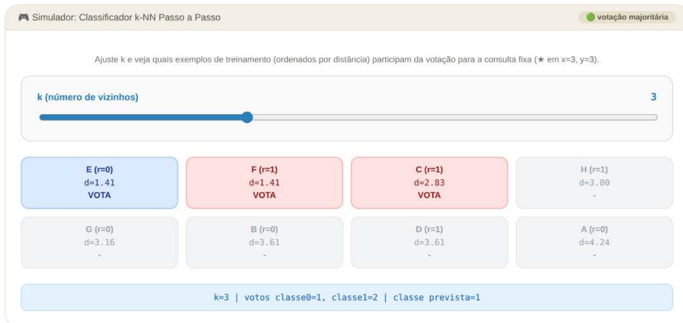
Figura 7.21: Simulador: Classificador k-NN Passo a Passo
