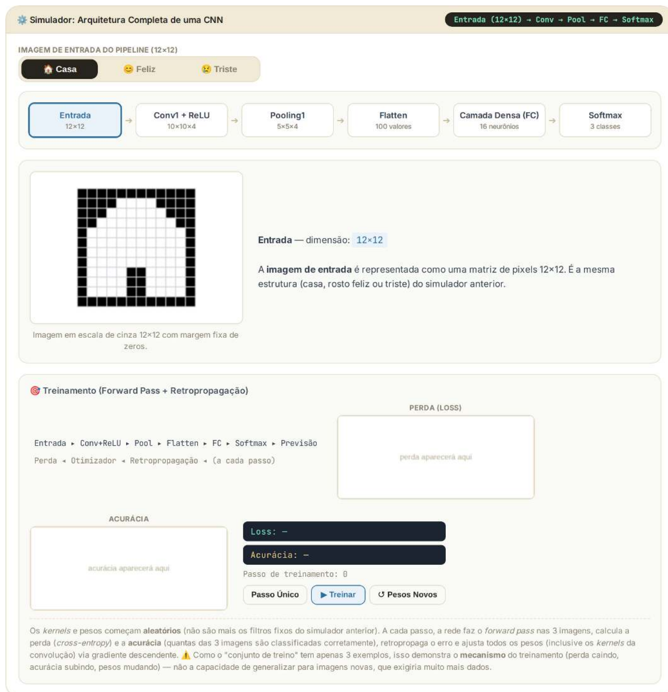
Figura 9.11: Simulador interativo da arquitetura de uma CNN: escolha uma das imagens de entrada 12 \times 12 (casa, rosto feliz ou triste), clique em cada bloco do pipeline — Entrada, Conv+ReLU , Pooling , Flatten , FC e Softmax — e execute passos de treinamento reais ( forward pass + retropropagação) para observar a perda e a acurácia evoluindo, os kernels sendo ajustados e o Softmax passando a apontar a classe correta.
