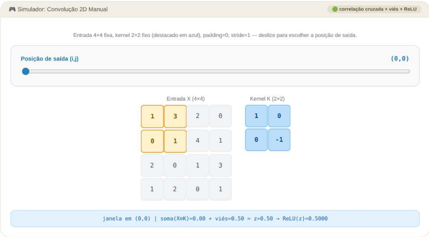
Figura 9.25: Simulador: Convolução 2D Manual (correlação cruzada + viés + ReLU)
