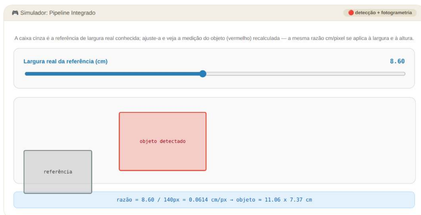
Figura 9.29: Simulador: Pipeline Integrado — NMS + Medição por Referência de Escala
