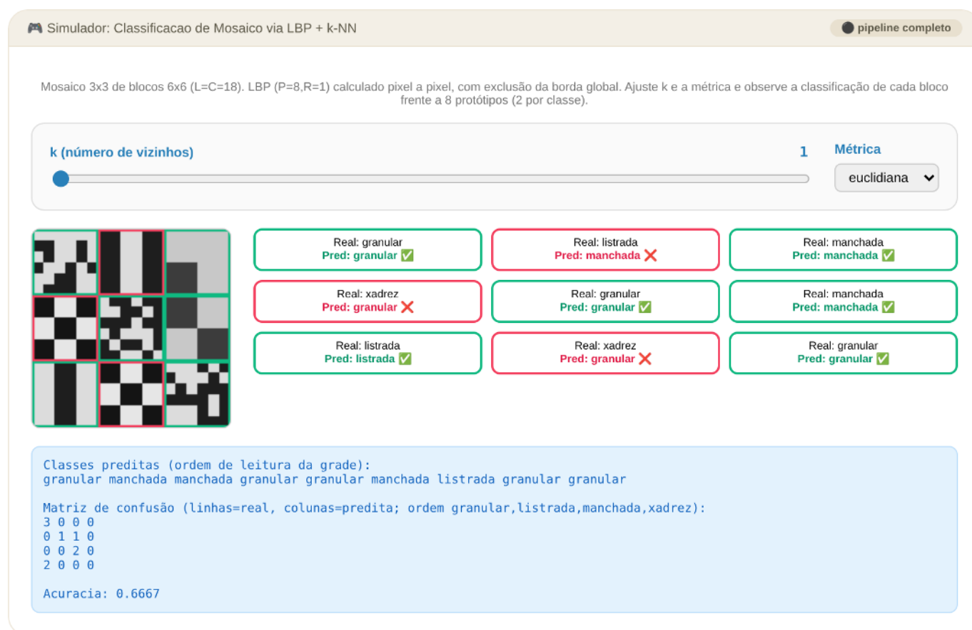
Figura 7.28: Simulador: Classificação de um Mosaico de Texturas via LBP + k-NN
