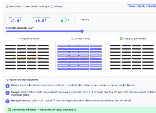
Figura 6.6: Simulador interativo de correção de inclinação ( deskew ): mova o slider para inclinar o documento e observe as três etapas do pipeline — imagem inclinada, bordas Canny e resultado corrigido.
