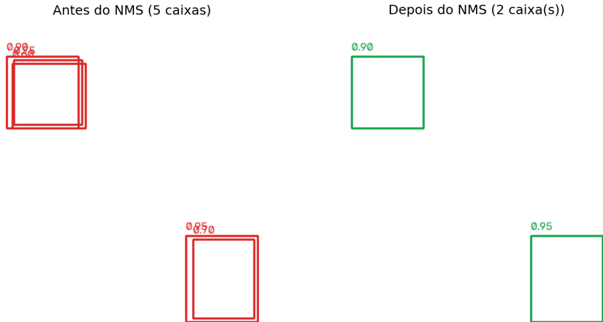
Figura 8.10: Efeito da Supressão de Não-Máximos (NMS): múltiplas detecções redundantes (esquerda) são reduzidas a uma detecção por objeto (direita).
