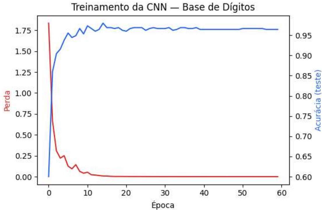
Figura 9.2: Curva de treinamento de uma CNN simples na base de dígitos: perda de treinamento e acurácia no conjunto de teste ao longo das épocas.
