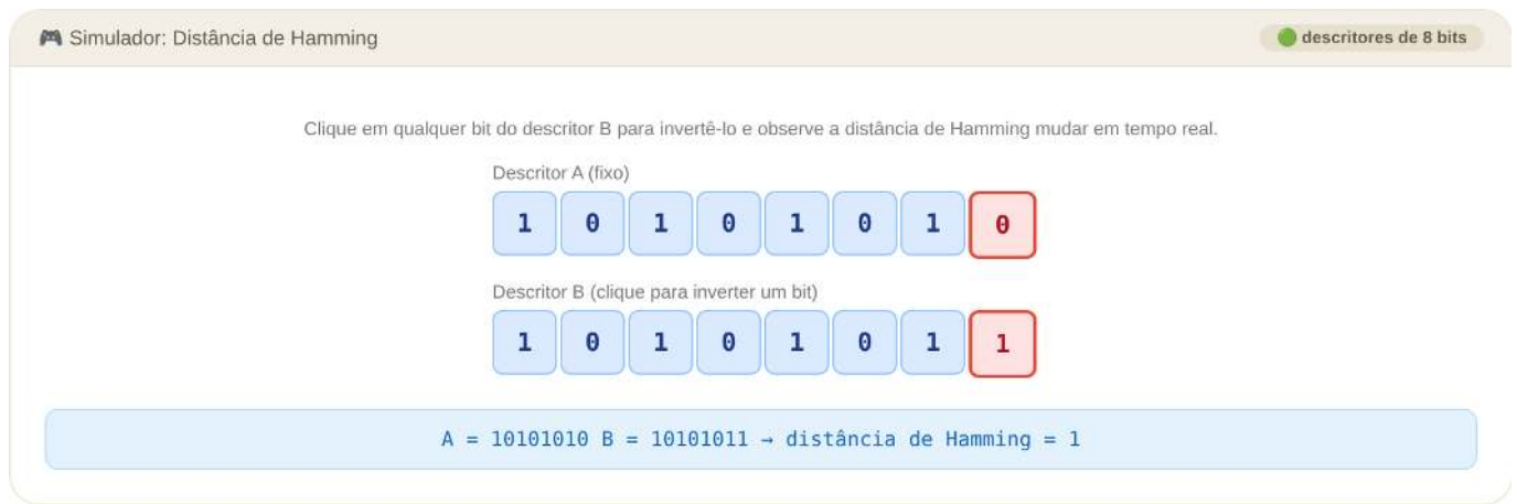
Figura 8.15: Simulador: Distância de Hamming entre Dois Descritores Binários
