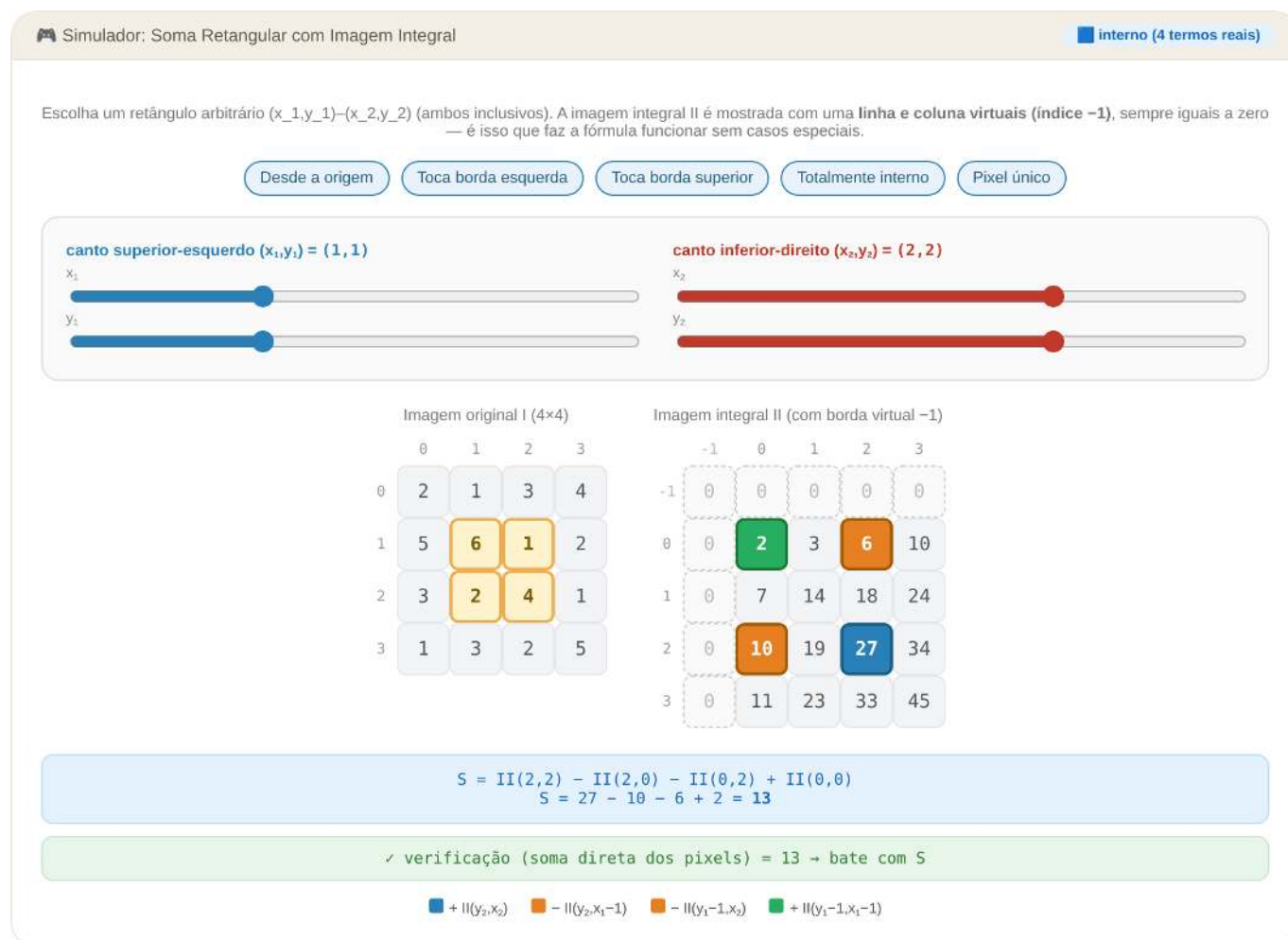
Figura 8.17: Simulador: Soma Retangular em O(1) — Múltiplas Situações de Borda
