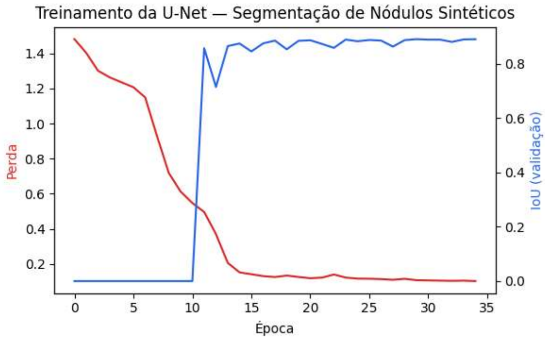
Figura 9.36: Evolução do treinamento da U-Net compacta: redução da perda e elevação do índice IoU médio no conjunto de validação ao longo de 35 épocas.
