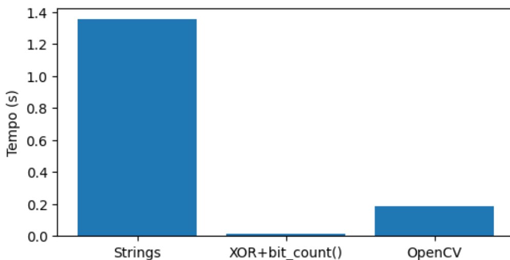
Figura 8.2: Comparação do desempenho de diferentes implementações da distância de Hamming.
