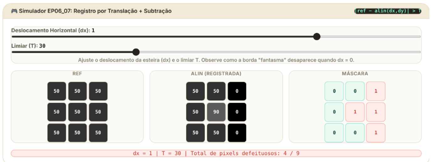
Figura 6.27: Simulador EP06_07: Pipeline de Inspeção — Registro por Translação e Subtração
