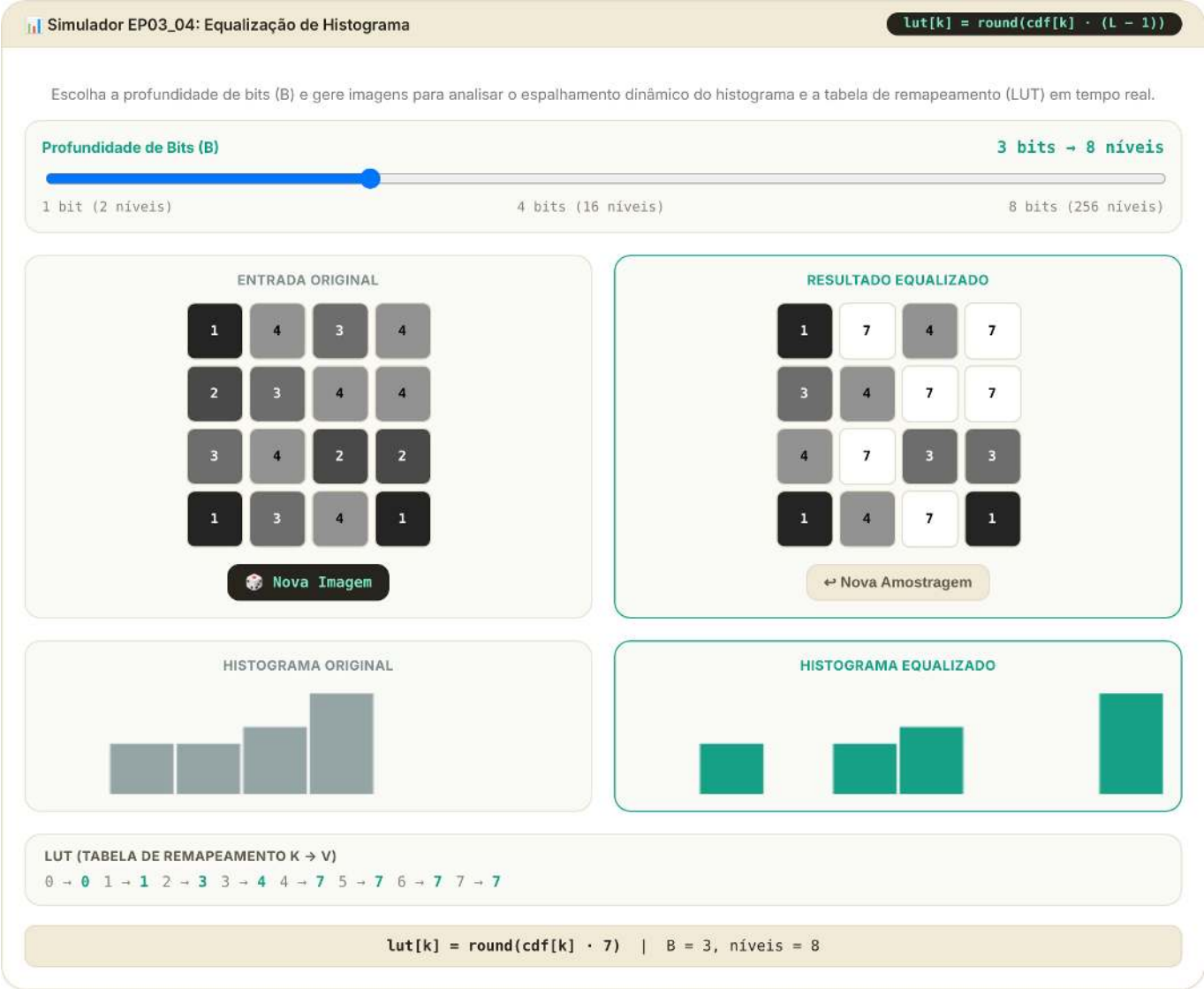
Versão interativa: https://fzampirolli.github.io/pdi-vc/simuladores/py.pt/cap03/sim-equalizacao.html Figura 3.29: Simulador EP03_04: Equalização de Histograma (Níveis L = 2^B )
