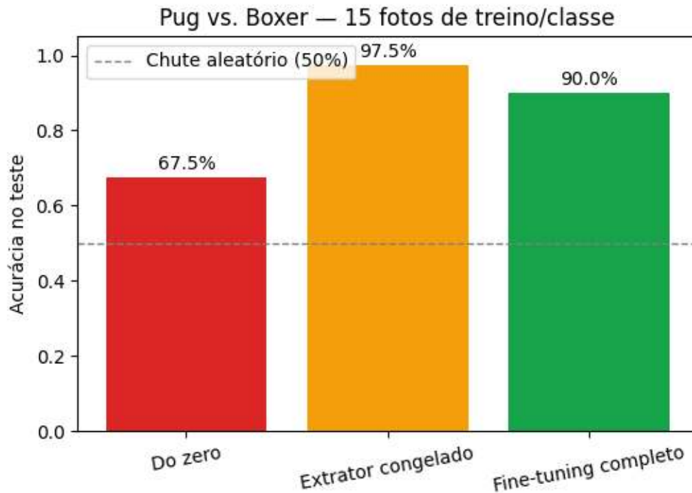
Figura 9.24: Comparação de acurácia no conjunto de teste real ( Pug vs. Boxer , 15 fotografias de treino por classe): do zero, extrator congelado e fine-tuning completo, todos sobre a mesma arquitetura ResNet-18.
