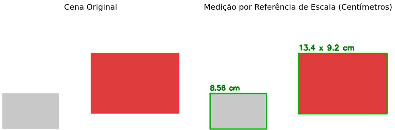
Figura 9.39: Medição de dimensões físicas reais utilizando um cartão de referência de escala conhecida (8,56 cm) renderizada via mm.show.
