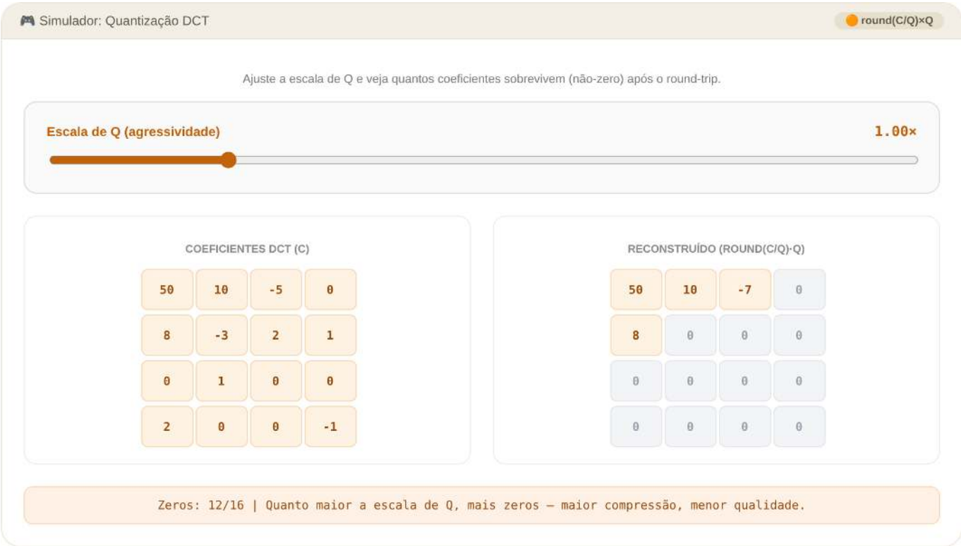
Figura 5.34: Simulador: Quantização DCT (round-trip)
