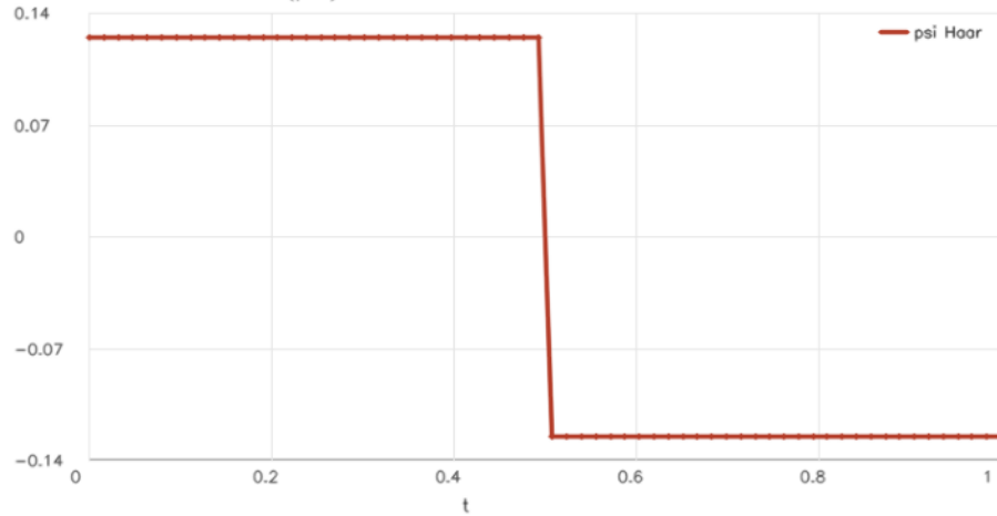
Ondaleta Haar (psi)
