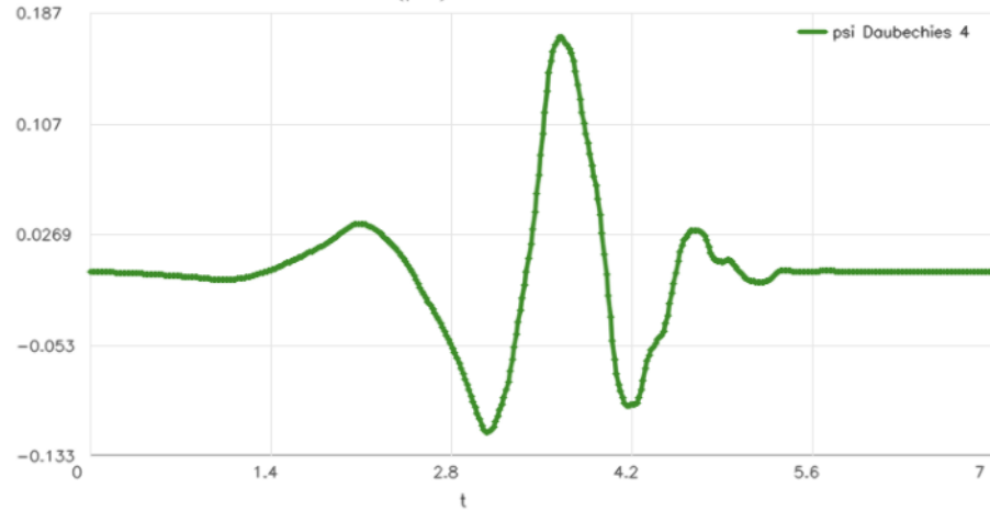
Ondaleta Daubechies 4 (psi)
