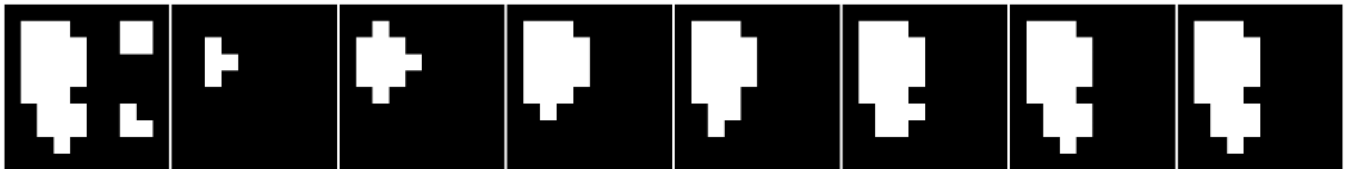
Figure 4.9: Pipeline de Reconstrução Morfológica por Dilatação Condicionada: a máscara contém dois objetos, o marcador isola apenas o núcleo do objeto principal, e as iterações reconstróem sua forma exata até a convergência.
