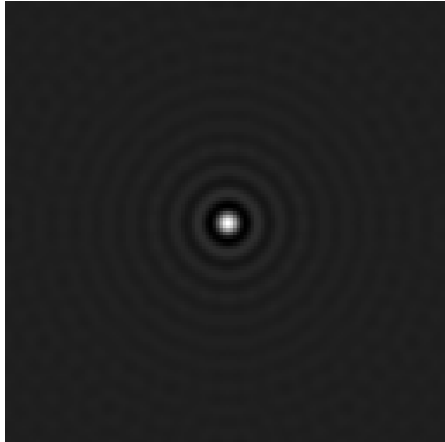
Espaco: ondulacoes da sinc (causa do ringing)
