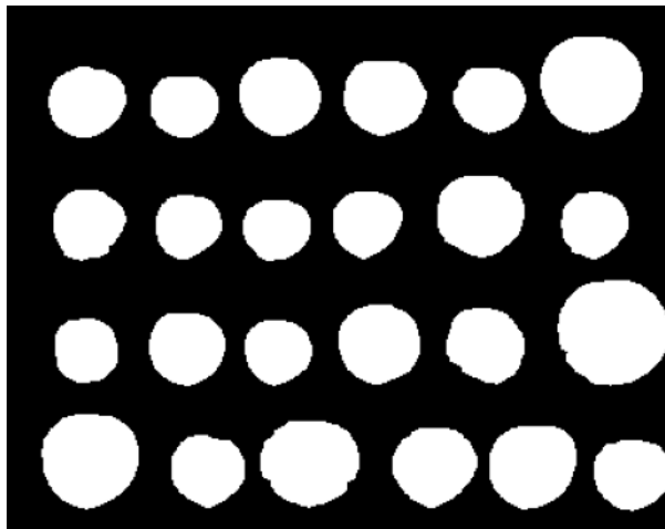
4. Apertura (limpieza)
