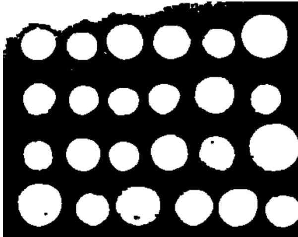
1. Umbralización (Otsu)
