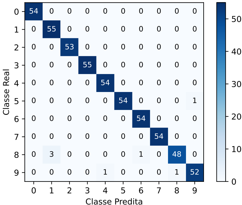
Matriz de Confusão — Pixels Brutos
