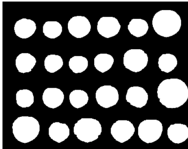
4. Ouverture (nettoyage)
