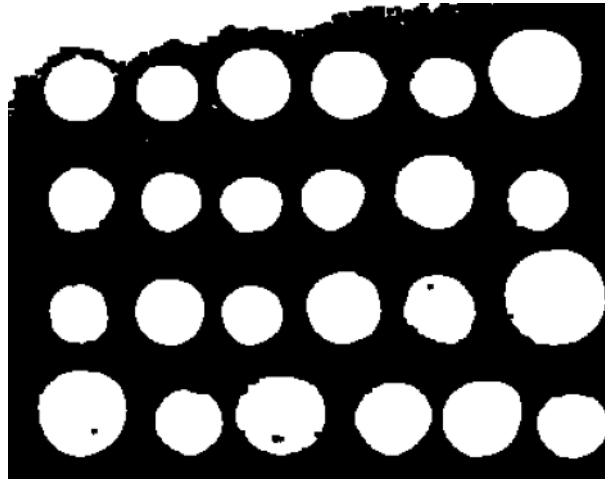
1. Seuillage (Otsu)
