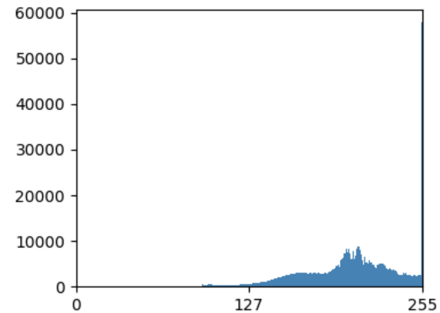
Istogramma - schiarita
