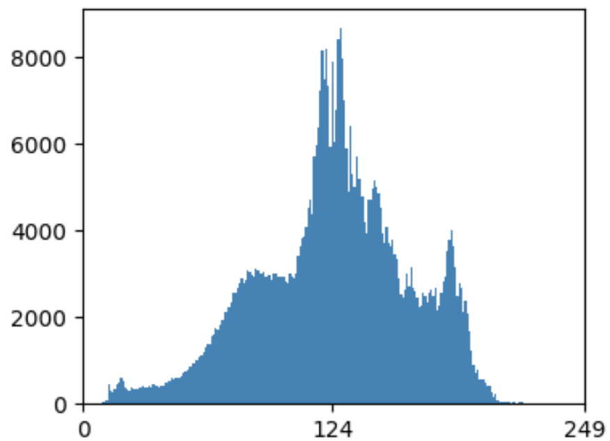
Istogramma - originale
