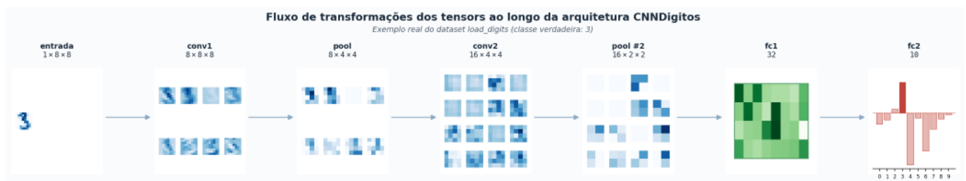
Figura 9.16: Fluxo de ativações da CNN treinada ao processar um exemplo real do dígito 3, do dataset load_digits : dimensões dos tensores camada a camada, da entrada ao logit de saída.
