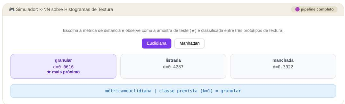
Figura 7.23: Simulador: Pipeline k-NN com escolha de metrica
