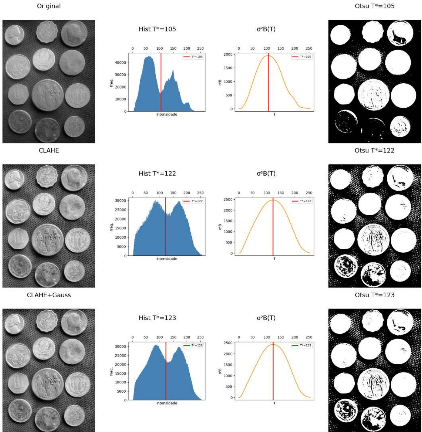
Figura 4.2: Comparação dos pré-processamentos: imagem | histograma+ T^* | \sigma^2_B(T) | Otsu. A melhor separação bimodal indica o limiar mais confiável.
