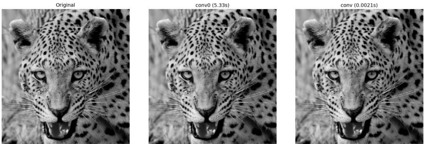
Figura 3.10: Correlação com kernel de média 3×3: versão didática (mm.conv0) vs. vetorizada (mm.conv via cv2.filter2D). A diferença máxima de 39 ocorre nas bordas.
