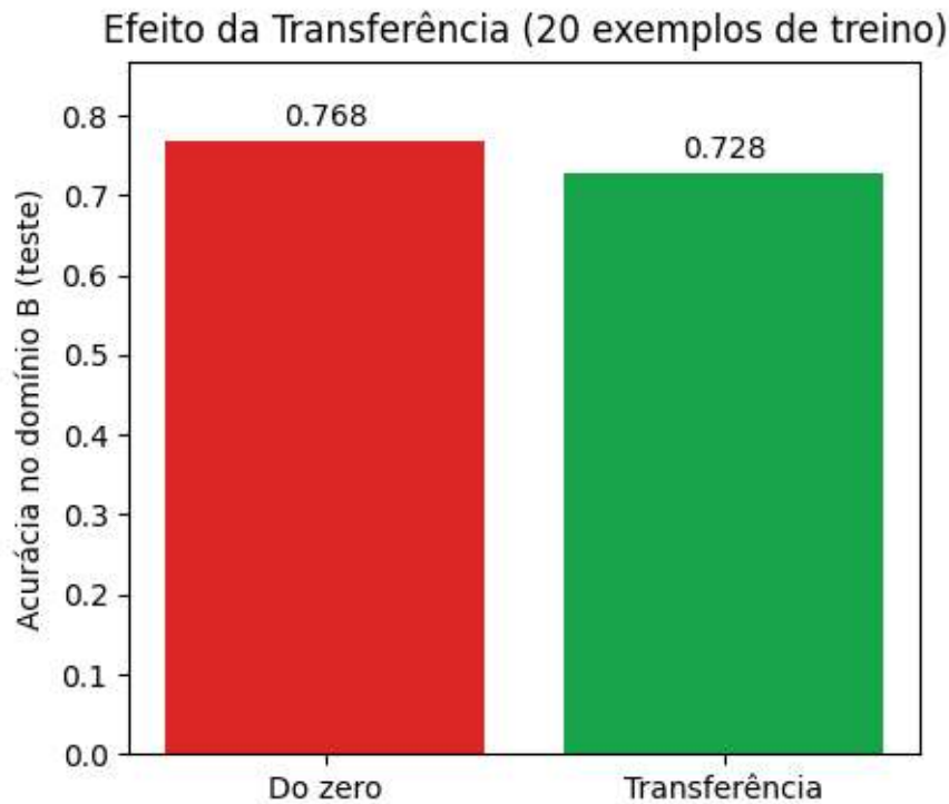
Figura 9.21: Comparação de acurácia no conjunto de teste do Domínio B (dígitos 5 a 9) sob restrição de dados (20 exemplos de treino): demonstração do impacto do congelamento rígido e da transferência negativa em redes de baixa capacidade.
