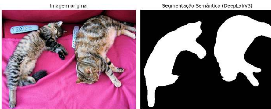
Figura 9.33: Mapa de segmentação semântica gerado pelo modelo DeepLabV3 pré-treinado: classificação pixel a pixel representada em matriz 2D exibida.
