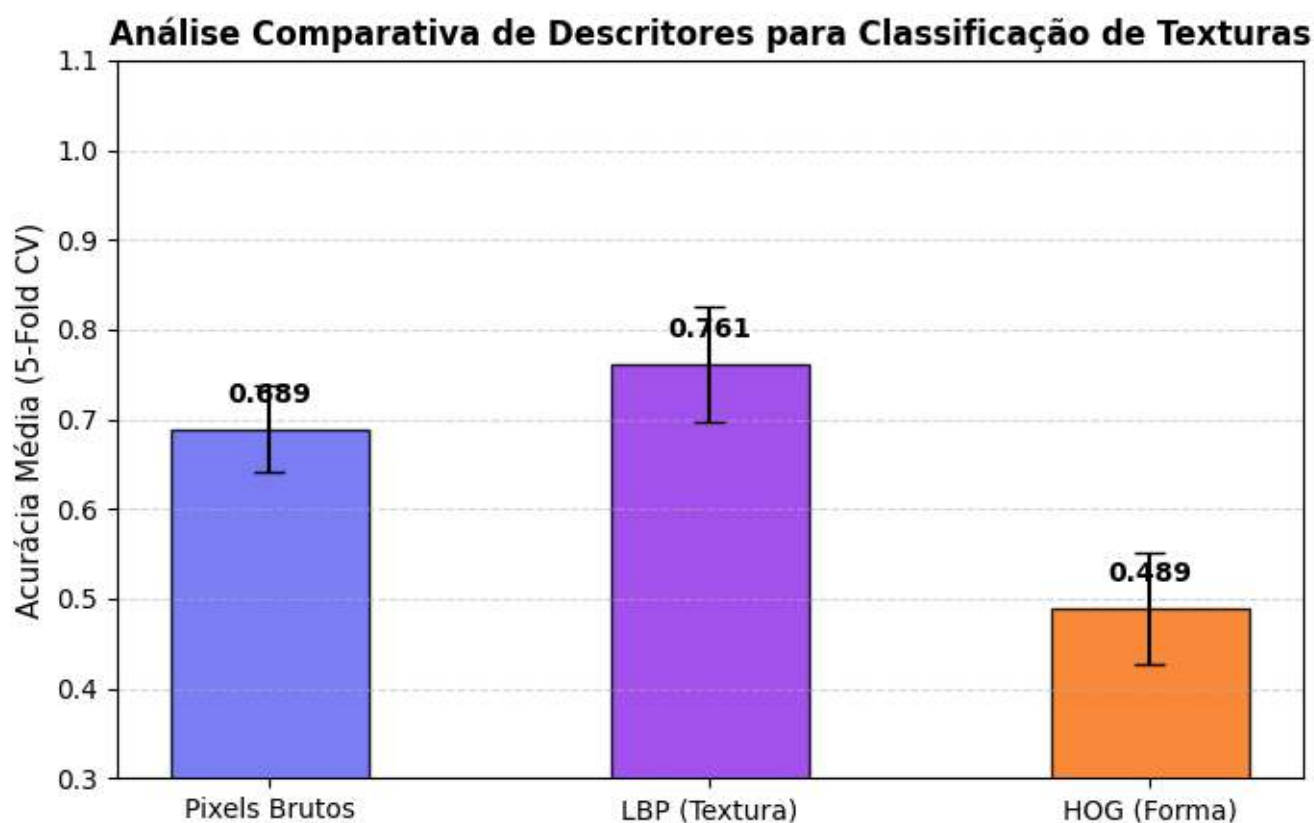
Figura 7.19: Acurácia média obtida via validação cruzada (5-fold) para os descritores de Pixels Brutos, LBP e HOG aplicados à base de texturas sintéticas.
