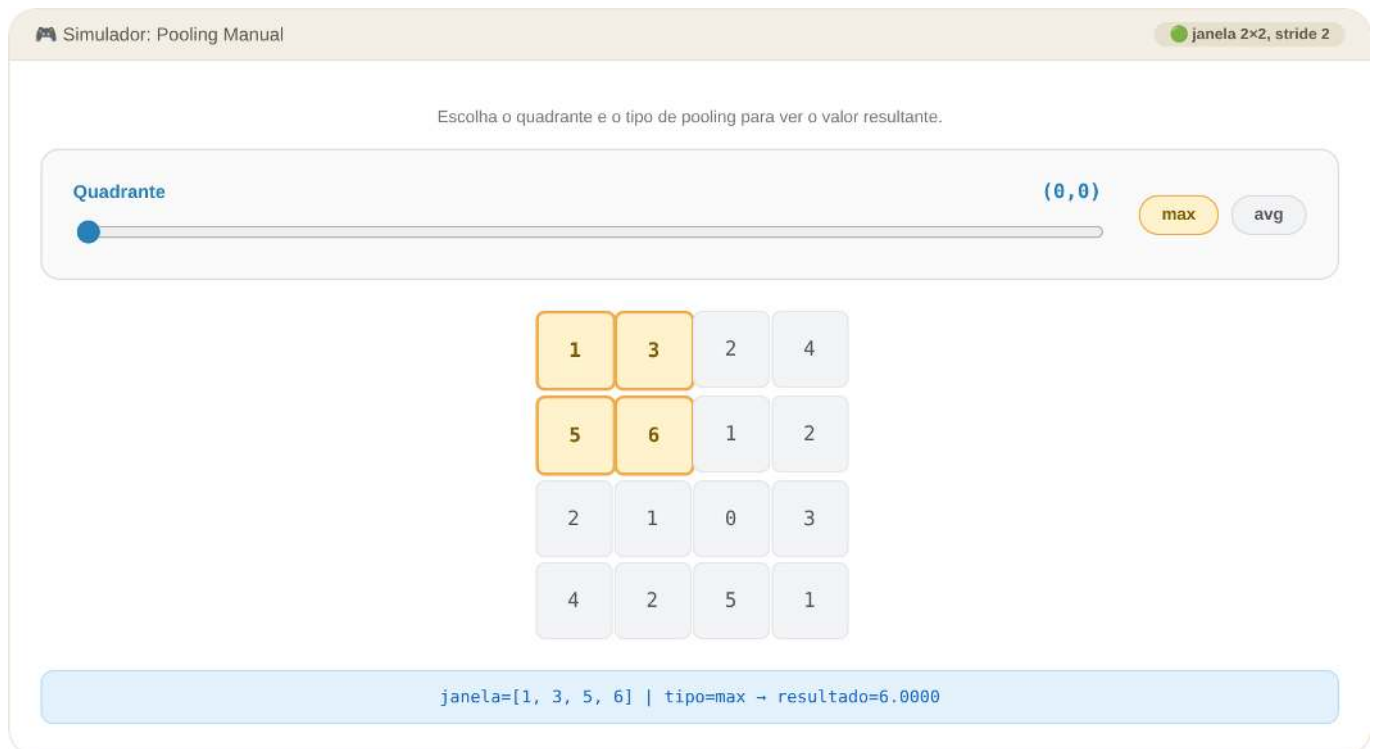
Figura 9.43: Simulador EP09_02: Pooling Manual (máximo vs. média)
