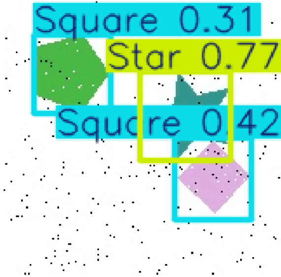
Figura 9.32: Comparação da inferência da YOLOv8 ajustada por transferência de aprendizado em uma imagem com ruído sal e pimenta e na versão restaurada pelo Filtro de Mediana. As caixas delimitadoras e classes previstas são exibidas sobre cada imagem.
