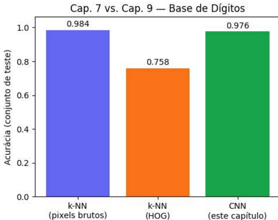
Figura 9.19: Comparação de acurácia entre os classificadores clássicos do Capítulo 7 (pixels brutos e HOG com k -NN) e a CNN treinada neste capítulo, na mesma base de dígitos.
