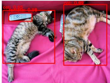
Figura 9.29: Resultado da inferência com o modelo Faster R-CNN pré-treinado no dataset COCO: identificação da classe, caixa delimitadora e pontuação de confiança sobrepostas.
