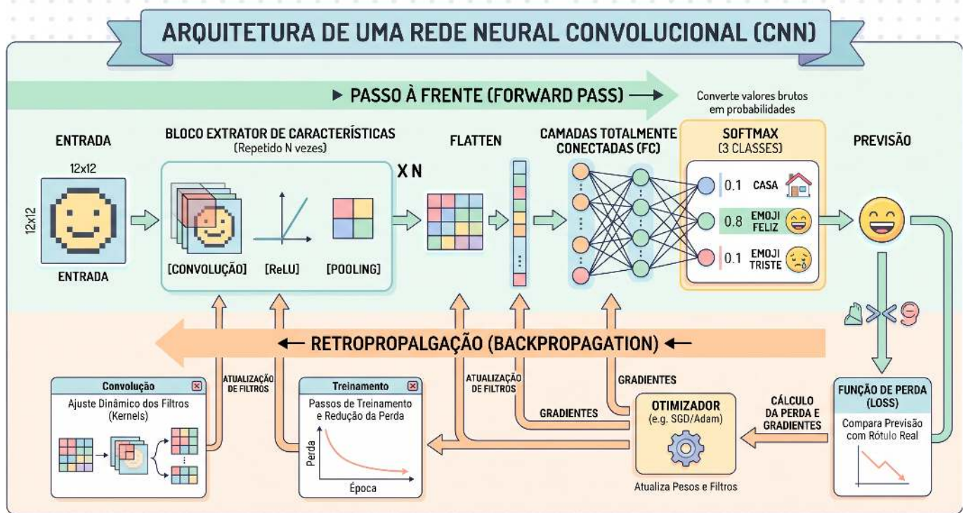
Figura 9.10: Arquitetura simplificada de uma CNN para classificação de imagens, destacando o forward pass e as etapas de treinamento por meio da função de perda, da retropropagação e do algoritmo de otimização.
