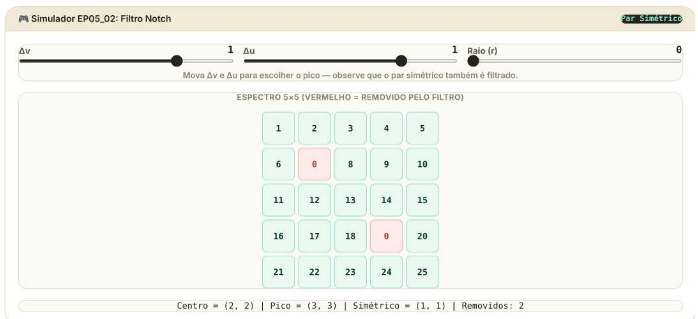
Figura 5.33: Simulador EP05_02: Filtro Notch
