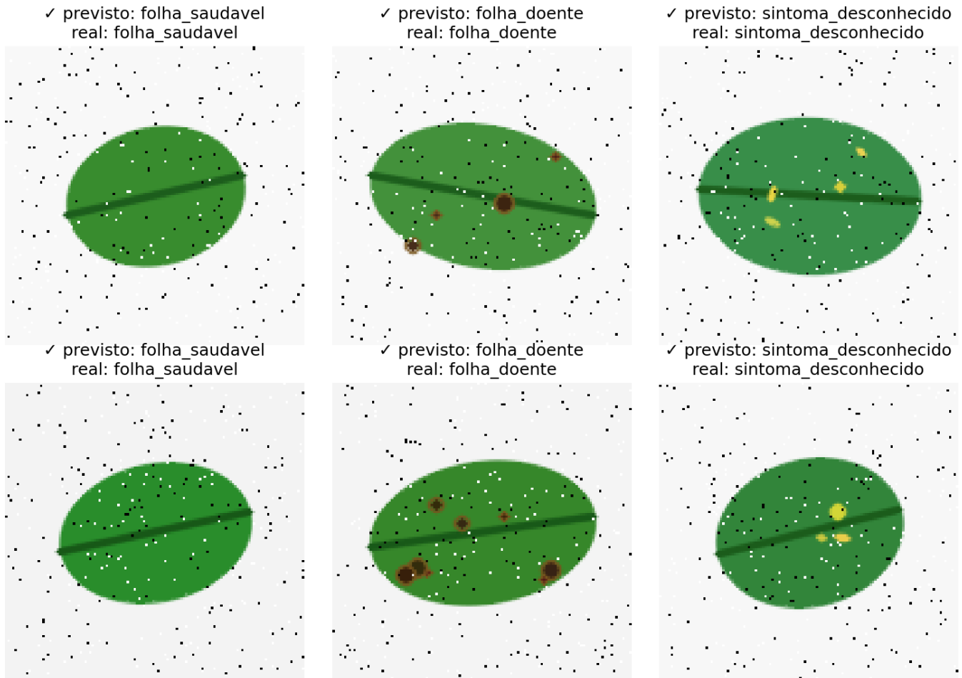
Figura 9.28: Predições da ResNet-18 ajustada em amostras de validação: rótulo previsto vs. rótulo real, com duas amostras por classe.
