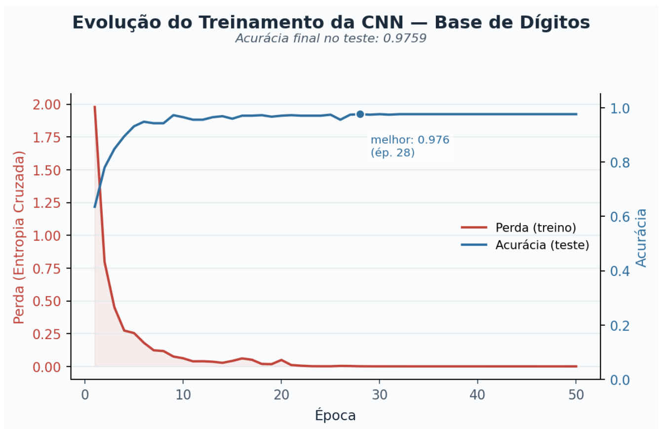
Figura 9.15: Curvas de treinamento e avaliação da CNN na base de dígitos: evolução da perda de entropia cruzada no conjunto de treinamento e da acurácia no conjunto de teste ao longo de 50 épocas.
