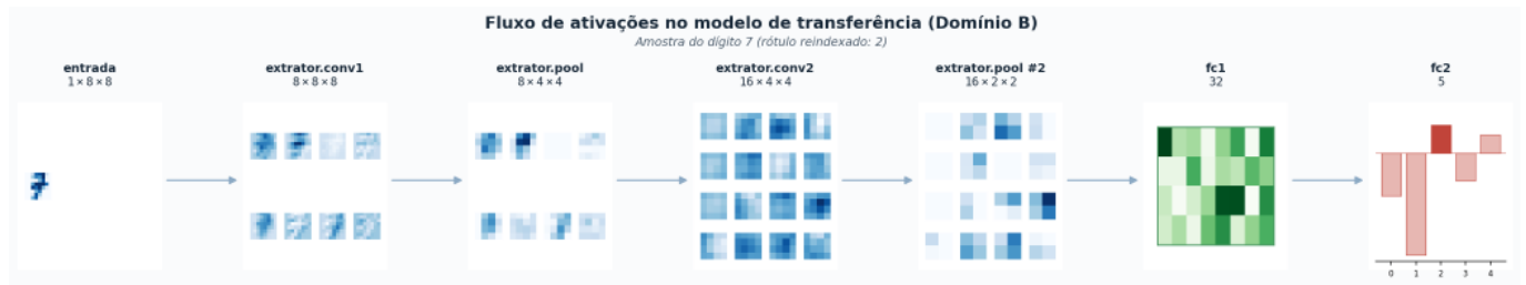
Figura 9.22: Fluxo de ativações e transformações dimensionais dos tensores no modelo de transferência de aprendizado ao processar uma amostra de teste do Domínio B (dígito 7, reindexado para classe 2).
