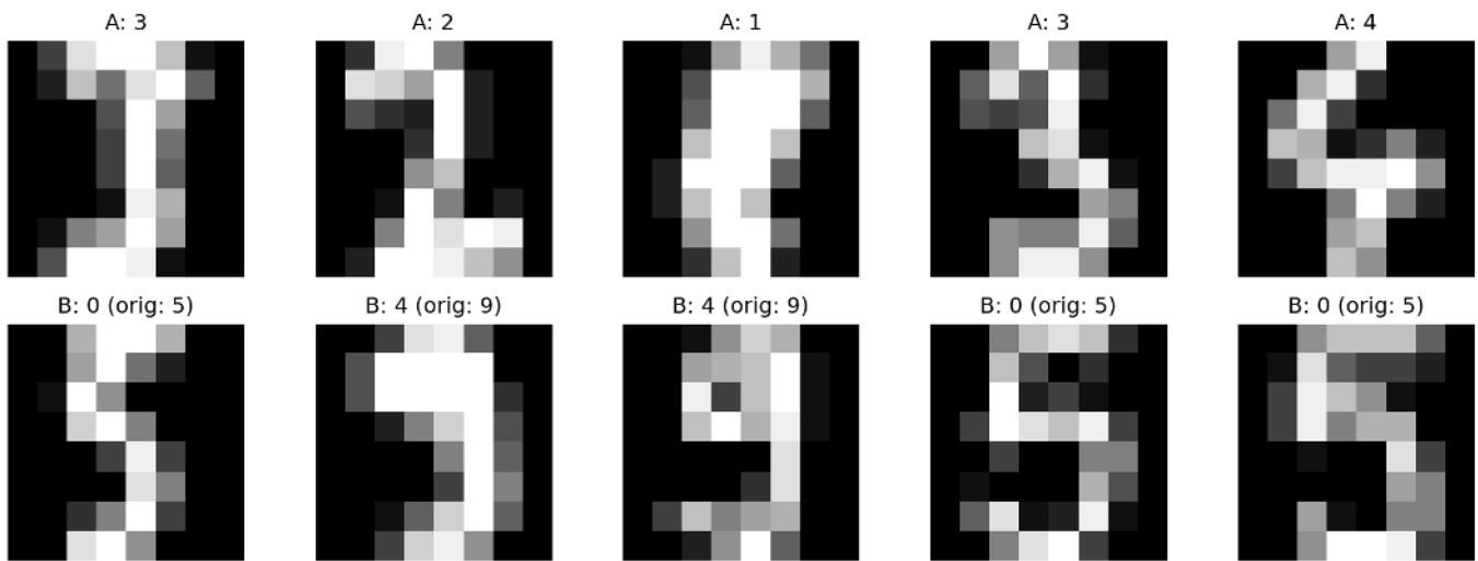
Figura 9.20: Amostras dos conjuntos de treinamento após pré-processamento e adequação dimensional aos tensores PyTorch: Domínio A (dígitos 0 a 4, tarefa de origem) e Domínio B (dígitos 5 a 9 reindexados para 0 a 4, tarefa de destino).
