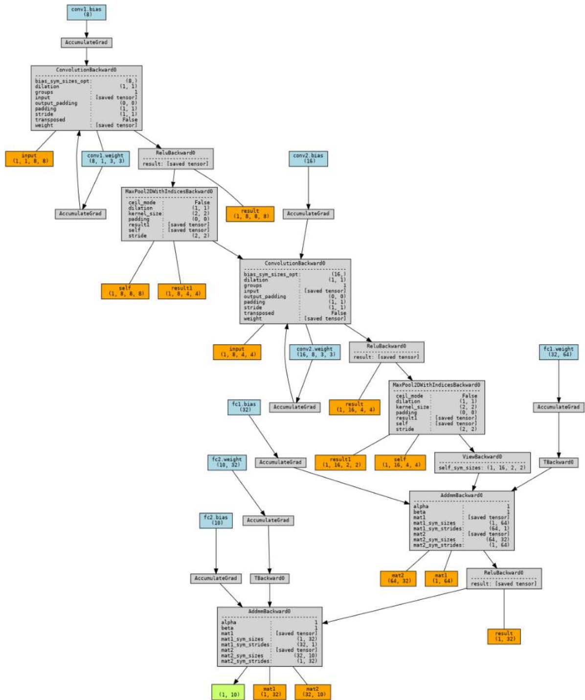
Figura 9.18: Grafo detalhado da classe CNNDigitos gerado via torchviz .
