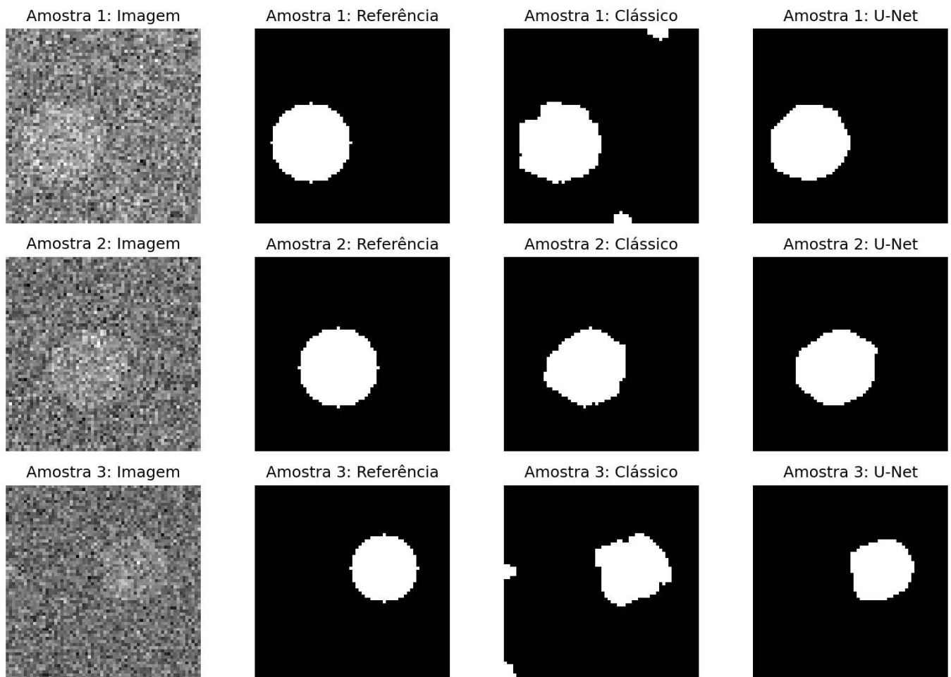
Figura 9.37: Comparativo quantitativo (IoU médio) e qualitativo entre a abordagem clássica e a U-Net treinada em três amostras de validação.
