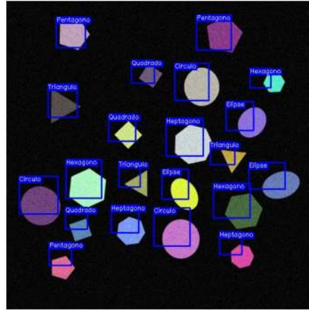
Figura 9.38: Inferência realizada por um modelo hospedado no Roboflow sobre uma imagem local. As detecções são retornadas em formato JSON e a imagem anotada é exibida para verificar rapidamente a qualidade do modelo antes da exportação do conjunto de dados para segmentação.
