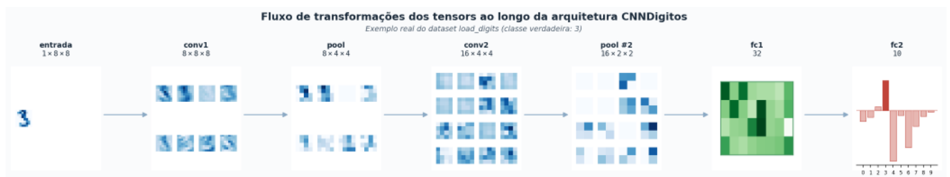
Figura 9.16: Fluxo de ativações da CNN treinada ao processar um exemplo real do dígito 3, do dataset load_digits : dimensões dos tensores camada a camada, da entrada ao logit de saída.
