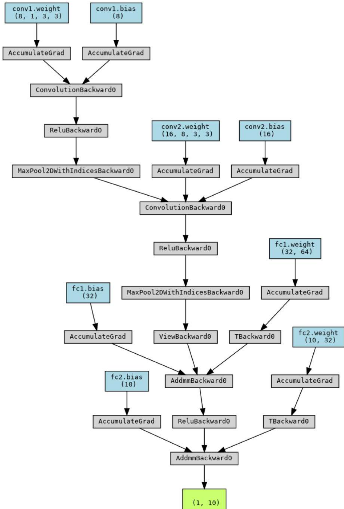
Figura 9.17: Grafo computacional da CNNDigitos gerado via torchviz , mostrando as operações de forward e os nós de gradiente ( backward ) associados a cada parâmetro treinável.
