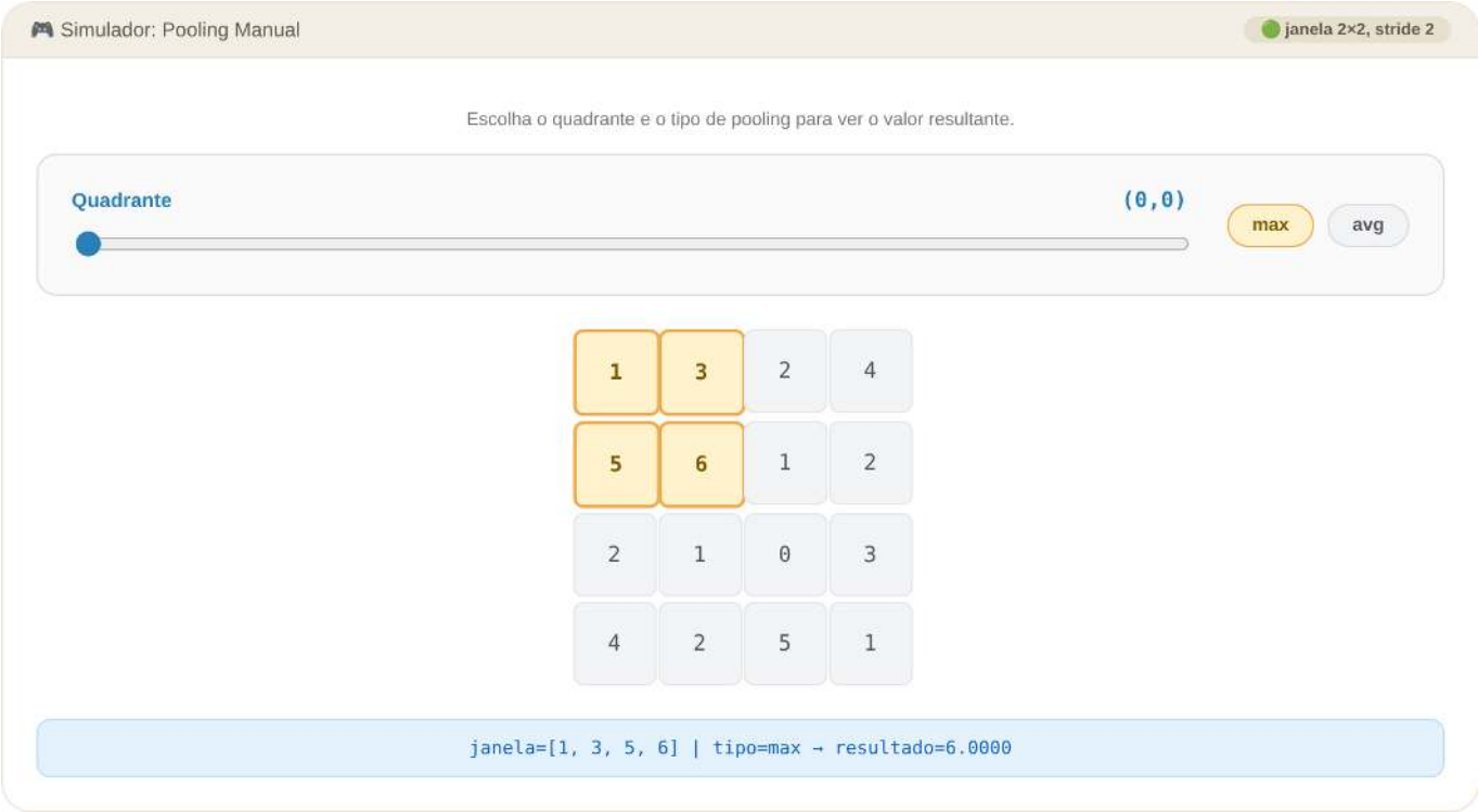
Figura 9.24: Simulador: Pooling Manual (máximo vs. média)
