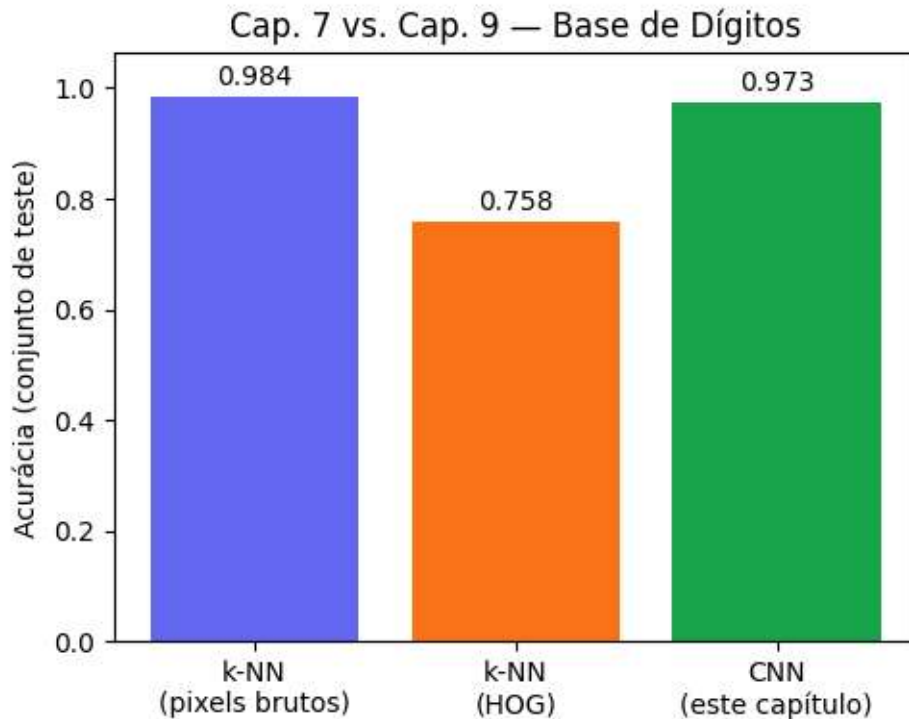
Figura 9.12: Comparação de acurácia entre os classificadores clássicos do Capítulo 7 (pixels brutos e HOG com k-NN) e a CNN treinada neste capítulo, na mesma base de dígitos.
