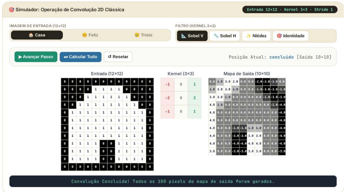
Figura 9.2: Simulador interativo de convolução 2D clássica: escolha entre as três imagens sintéticas de entrada 12x12 (casa, rosto feliz ou triste) e um filtro 3x3 (Sobel V, Sobel H, Nitidez ou Idêntidade) e avance passo a passo para observar como os produtos internos locais do campo receptivo constroem o mapa de características célula a célula.
