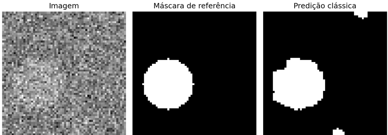
Figura 9.17: Linha de base clássica de segmentação: borrão gaussiano, limiarização de Otsu e abertura morfológica, aplicados a uma imagem de validação.
