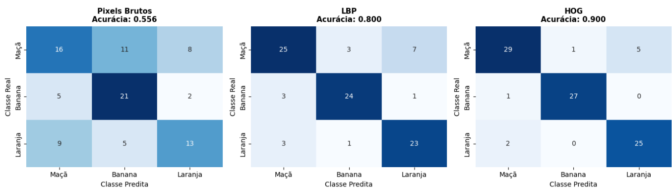
Figura 7.6: Matrizes de confusão obtidas pelo classificador k-NN utilizando três descritores diferentes. As linhas representam a classe real (Maçã, Banana e Laranja) e as colunas a classe predita. Quanto maior a concentração de valores na diagonal principal, melhor o desempenho do descritor.
