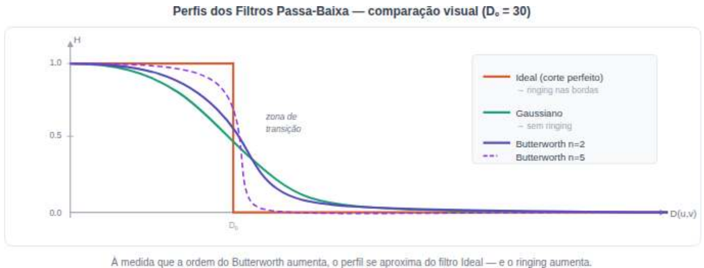
Figura 5.11: Filtros passa-baixa.
