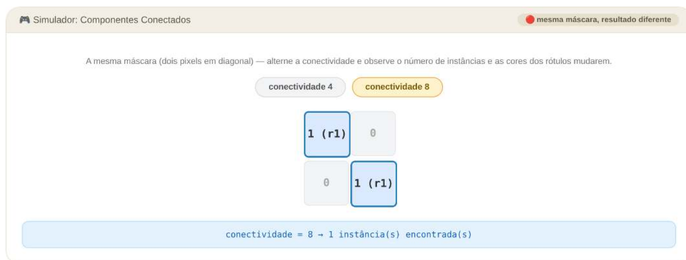
Figura 8.18: Simulador: Rotulagem de Componentes Conectados — Conectividade 4 vs. 8
