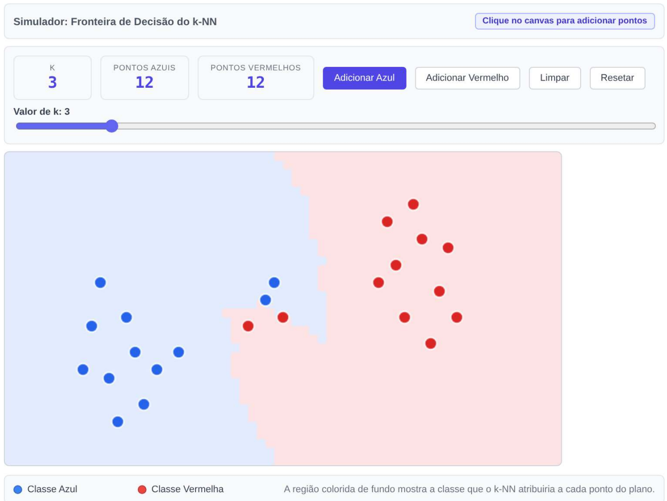
Figura 7.10: Simulador interativo da fronteira de decisão do k-NN: adicione pontos de treinamento e ajuste o valor de k para observar o efeito sobre a região de decisão.
