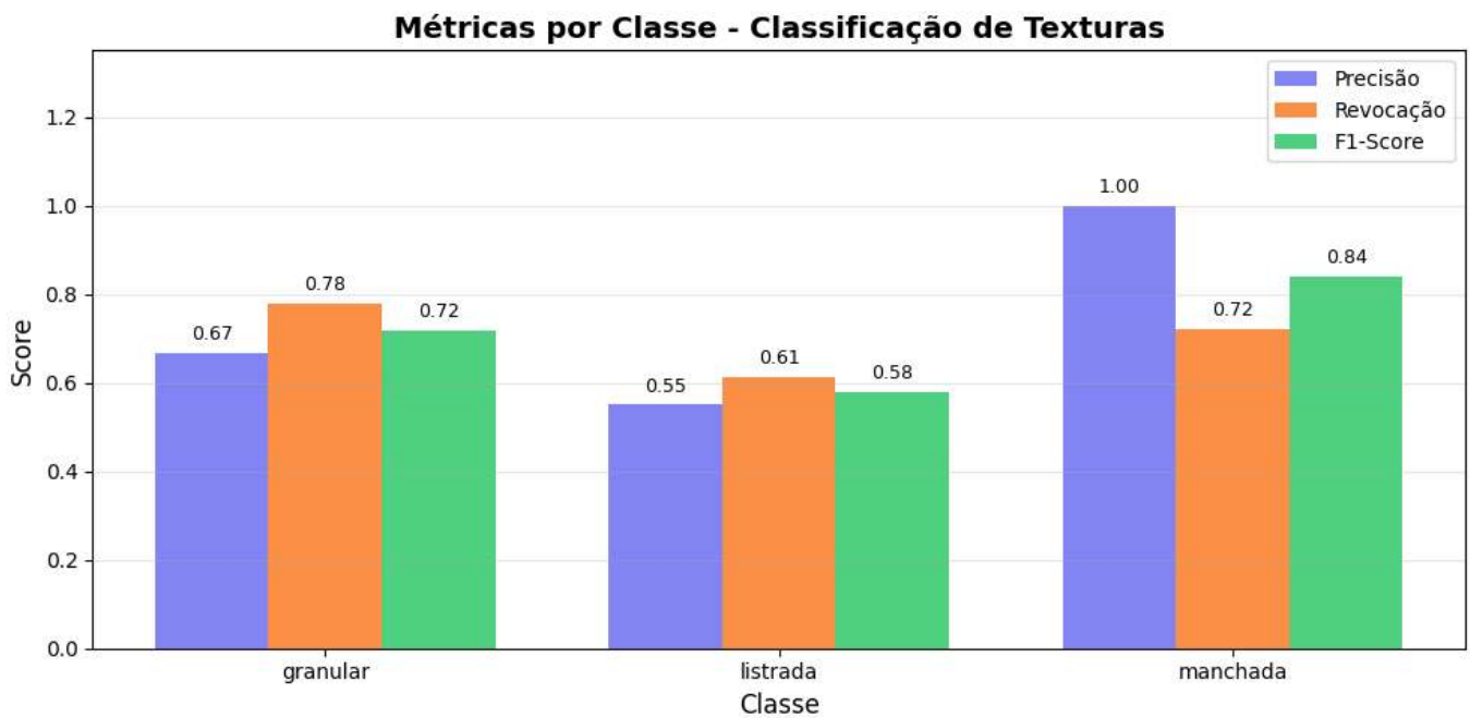
Figura 7.18: Métricas de avaliação detalhadas para o classificador k -NN com descritores LBP
