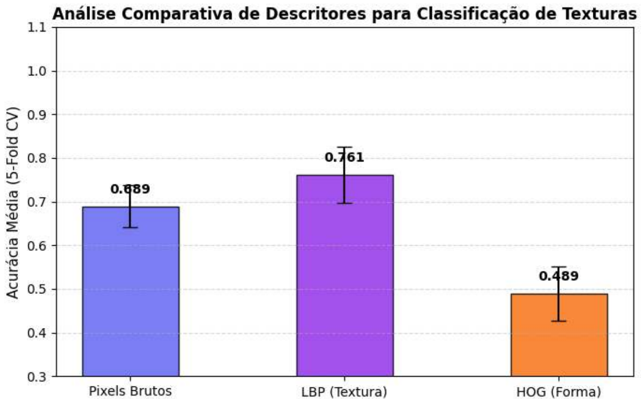
Figura 7.17: Acurácia média obtida via validação cruzada (5-fold) para os descritores de Pixels Brutos, LBP e HOG aplicados à base de texturas sintéticas.
