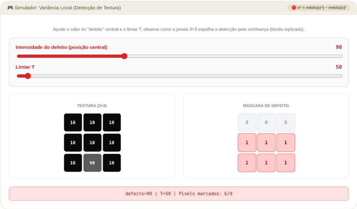
Figura 6.26: Simulador: Mapa de Variância Local para Detecção de Textura
