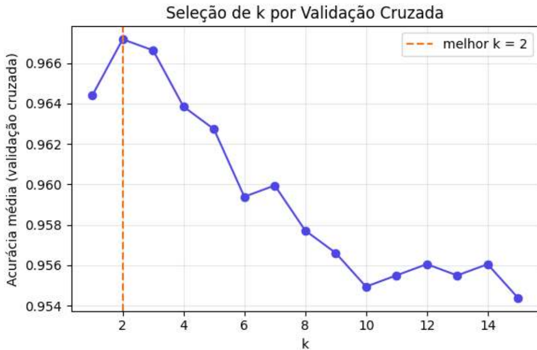
Figura 7.14: Acurácia média por validação cruzada (5 partições) em função do parâmetro k , para a base de dígitos com vetores de intensidade brutos.
