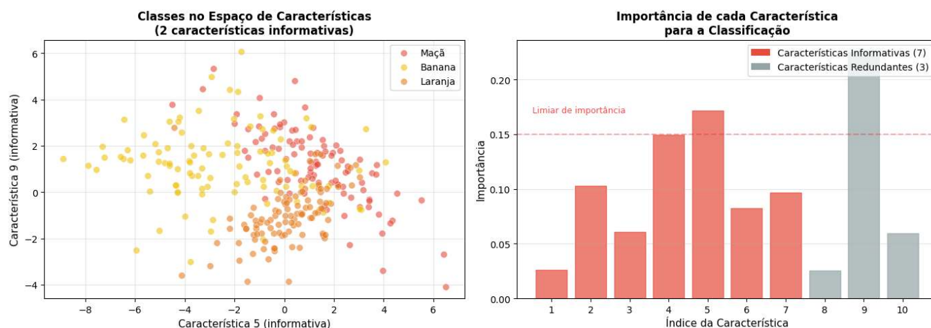
Figura 7.8: Ilustração do processo de geração de dados sintéticos com make_classification . À esquerda, visualização das três classes em um espaço bidimensional formado por duas características informativas. À direita, importância relativa de cada característica para a classificação, evidenciando que apenas 7 das 10 características são efetivamente discriminativas, enquanto as demais são redundantes (2) ou repetidas (1).
