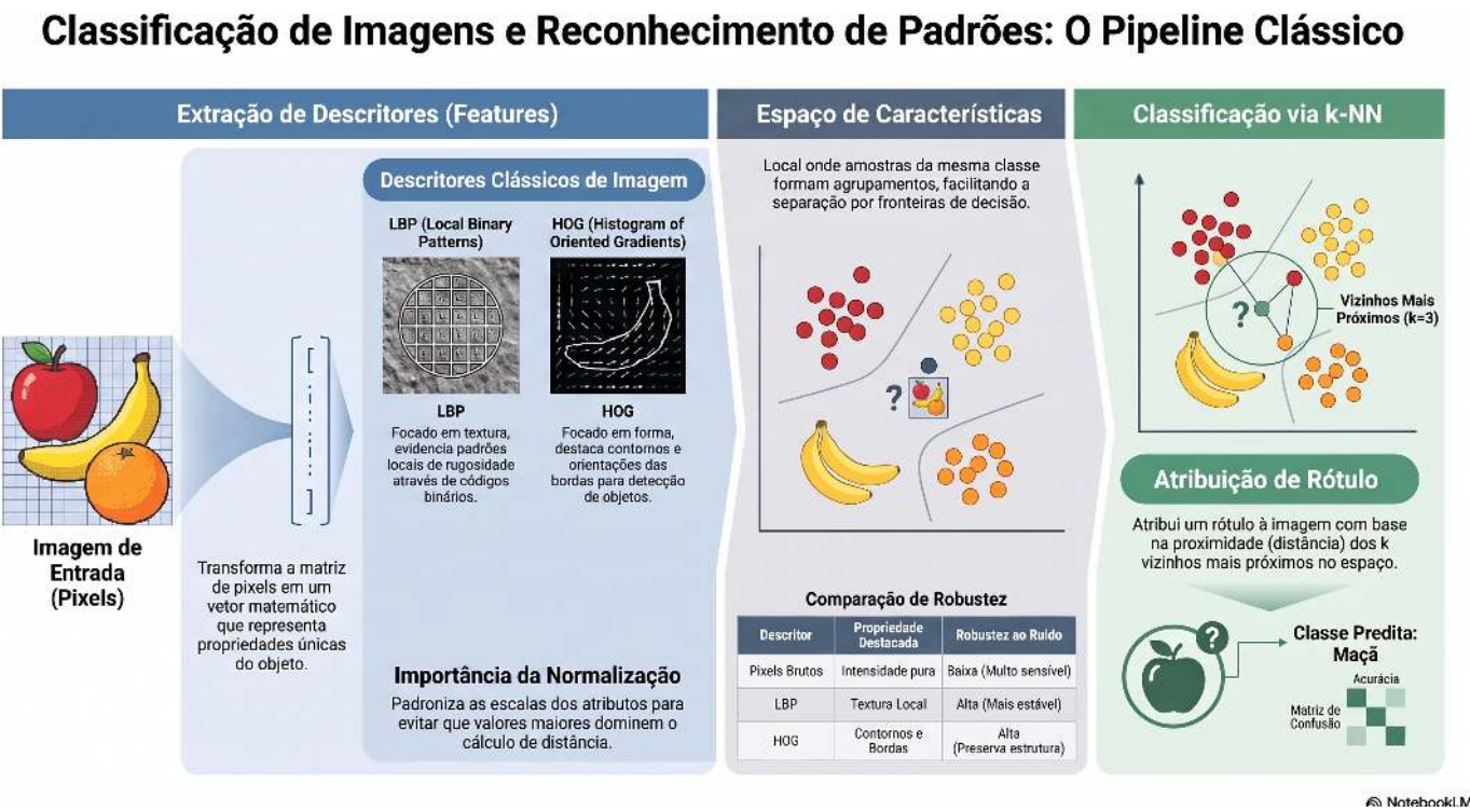
Figura 7.2: Panorama do pipeline clássico de classificação de imagens: extração de descritores (LBP, HOG), formação do espaço de características e classificação via k-NN. Não se aplica a modelos de deep learning (CNNs, YOLO), que aprendem features end-to-end diretamente dos pixels. Fonte: elaborado com auxílio do Gemini Notebook (Google, 2025).
