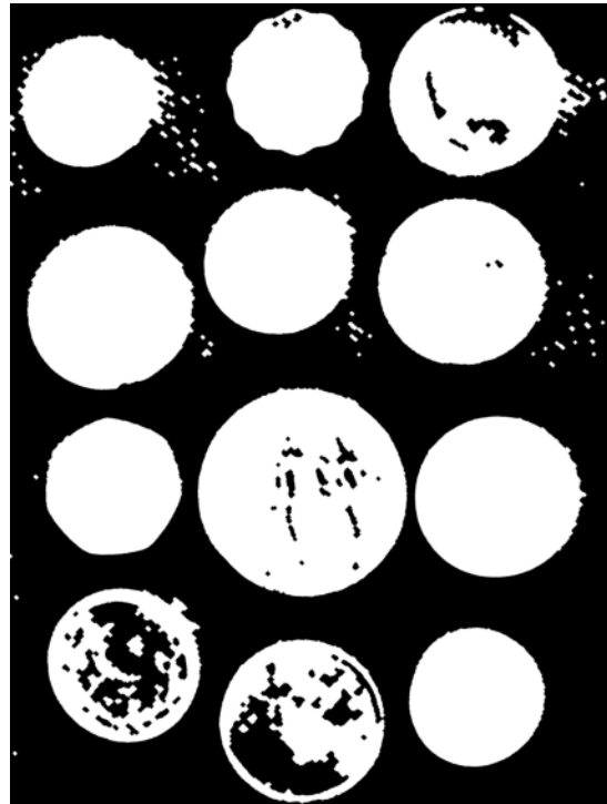
ASF-OC (n=7)
