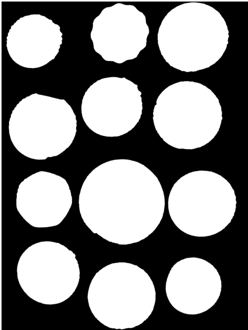
Segmentation finale
