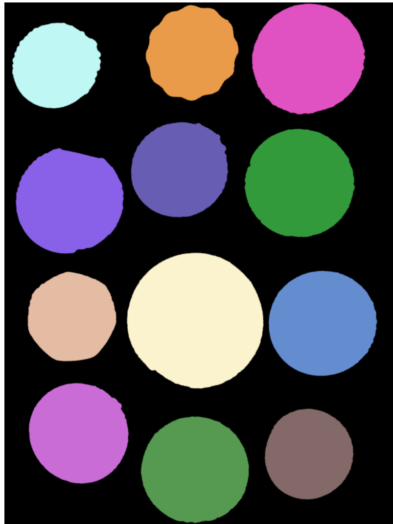
Composants connexes
