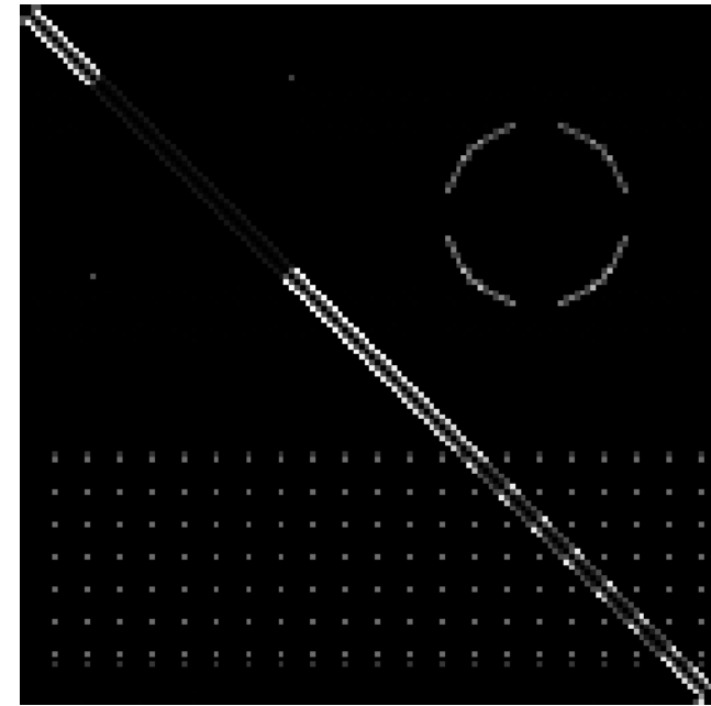
bior2.2 — HH 1
