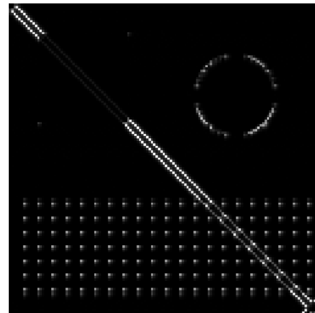
db4 — HH 1
