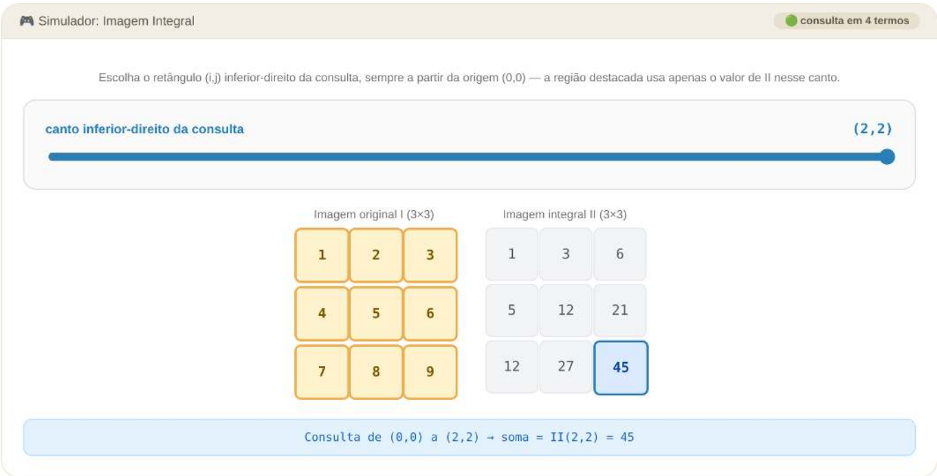
Figura 8.12: Simulador: Imagem Integral e Consulta Retangular em O(1)
