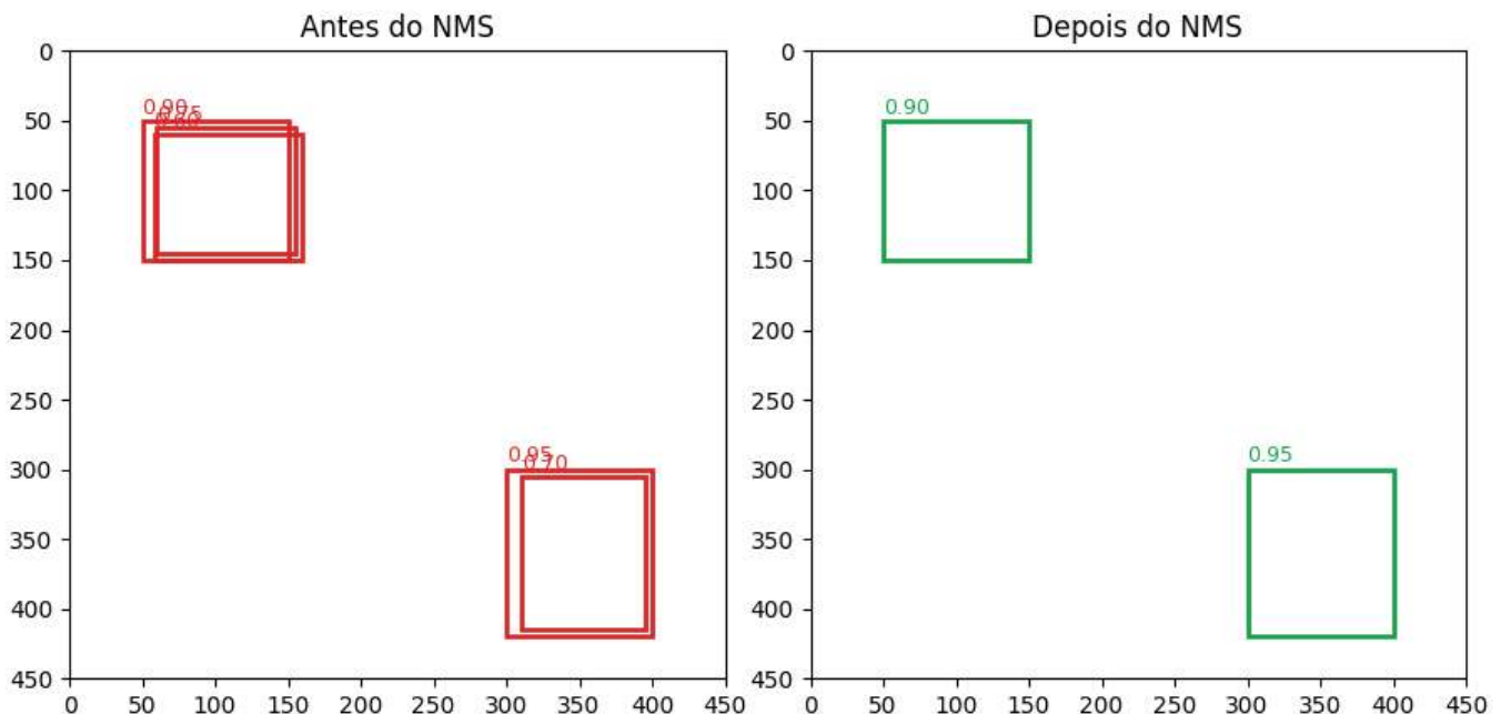
Figura 8.8: Efeito da Supressão de Não-Máximos (NMS): múltiplas detecções redundantes (esquerda) são reduzidas a uma detecção por objeto (direita).
