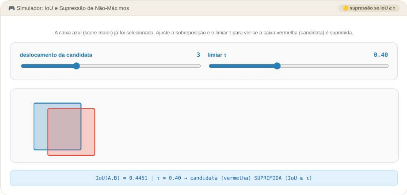
Figura 8.13: Simulador: IoU e Supressão de Não-Máximos
