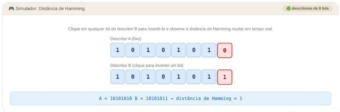
Figura 8.10: Simulador: Distância de Hamming entre Dois Descritores Binários
