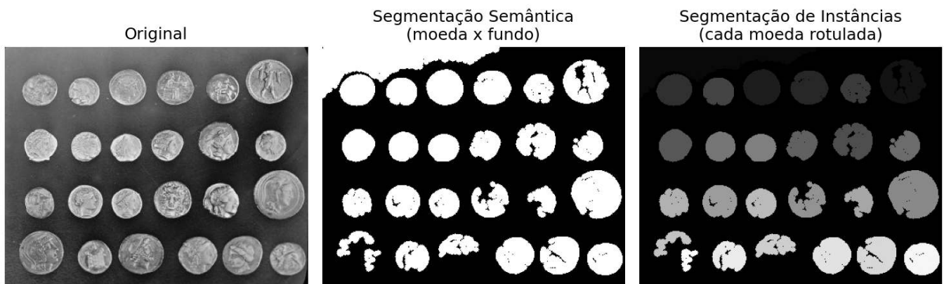
Figura 8.9: Segmentação clássica (não baseada em aprendizado profundo): máscara semântica (moeda x fundo) via limiarização de Otsu, e segmentação de instâncias via rotulagem de componentes conectados.
