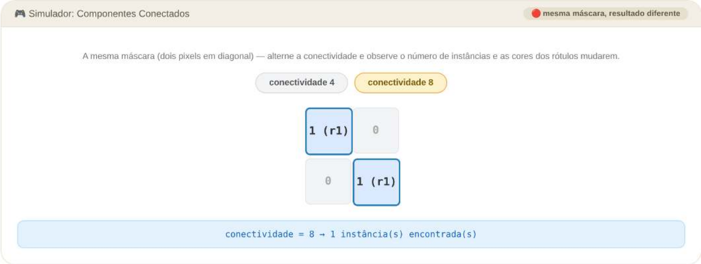
Figura 8.14: Simulador: Rotulagem de Componentes Conectados — Conectividade 4 vs. 8
