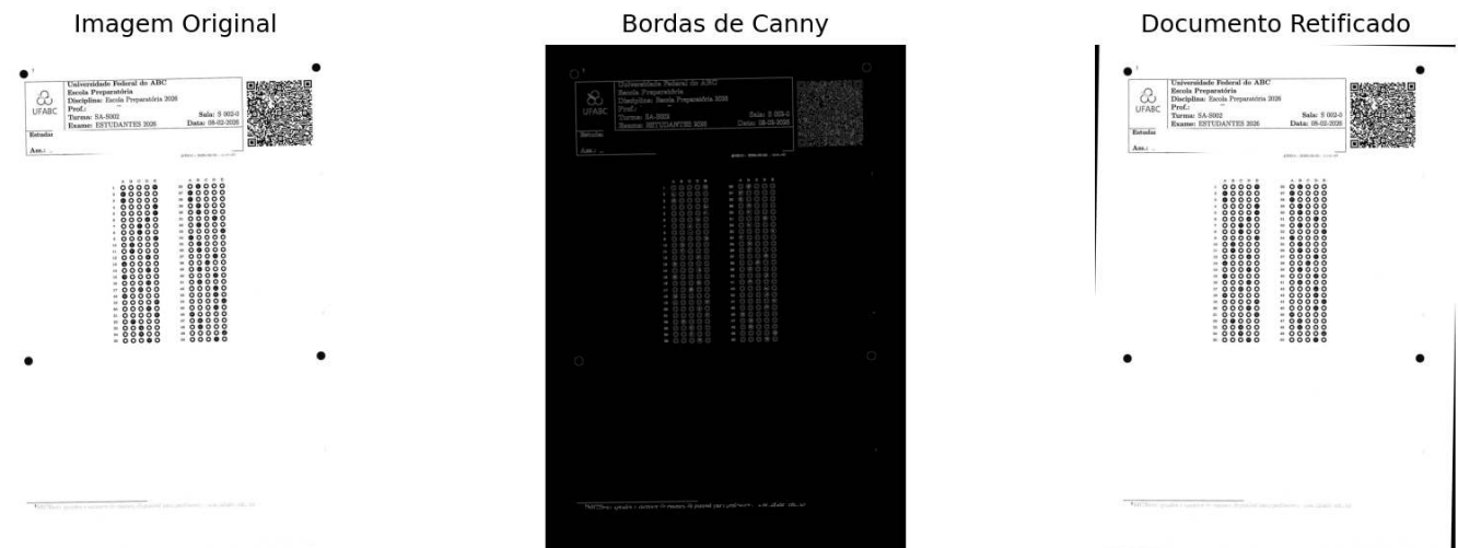
Figura 6.4: Pipeline de retificação axial: exibição comparativa entre a entrada rotacionada original, o mapa de gradientes estruturais de Canny e o resultado final alinhado com fundo normalizado em branco.
