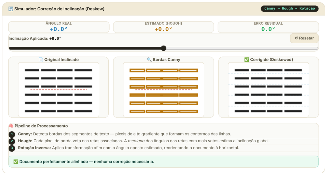
Figura 6.6: Simulador interativo de correção de inclinação ( deskew ): mova o slider para inclinar o documento e observe as três etapas do pipeline — imagem inclinada, bordas Canny e resultado corrigido.
