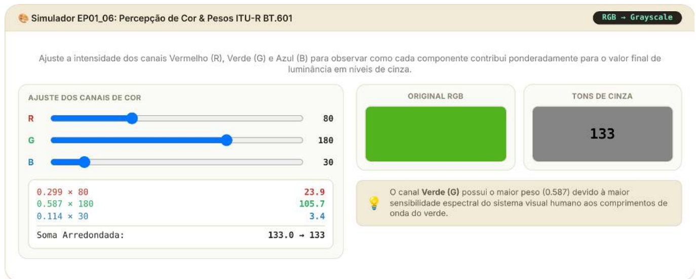
Figura 1.17: Simulador EP01_06: Conversão RGB para Grayscale (Ponderação Perceptual ITU-R BT.601)
