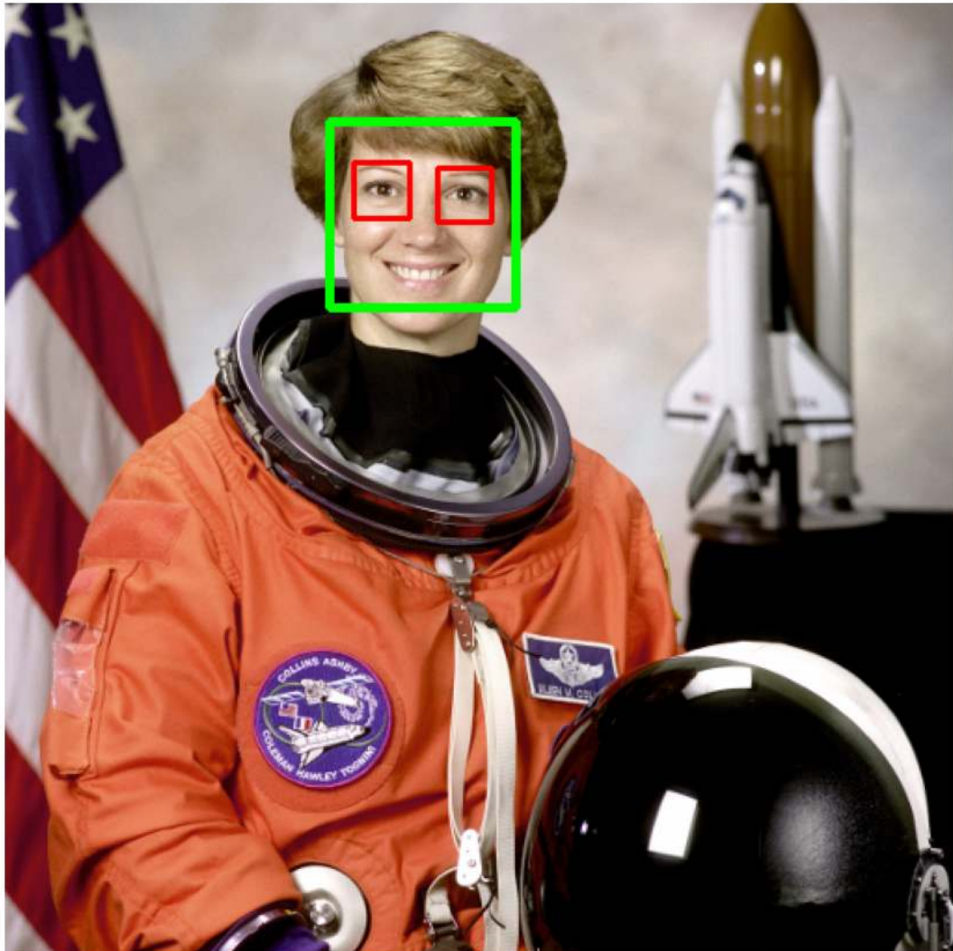
Figura 8.5: Detecção de faces e olhos com Haar Cascade na imagem astronaut (scikit-image).
