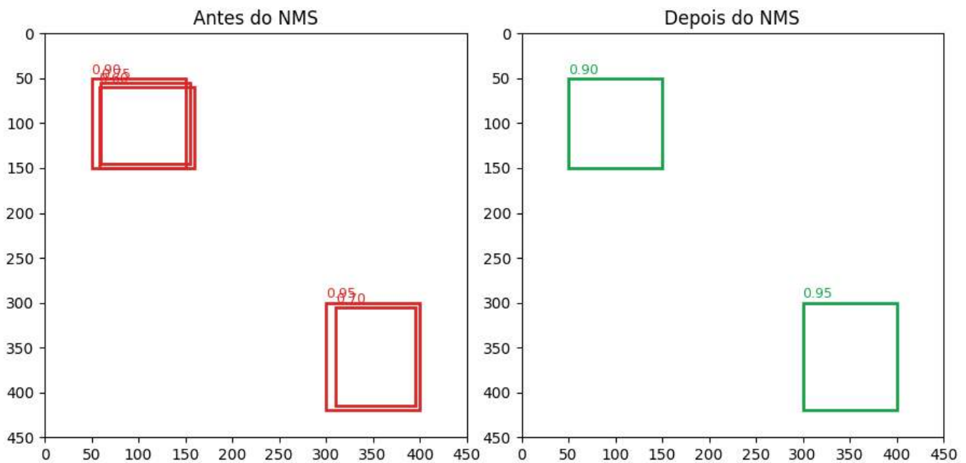
Figura 8.6: Efeito da Supressão de Não-Máximos (NMS): múltiplas detecções redundantes (esquerda) são reduzidas a uma detecção por objeto (direita).
