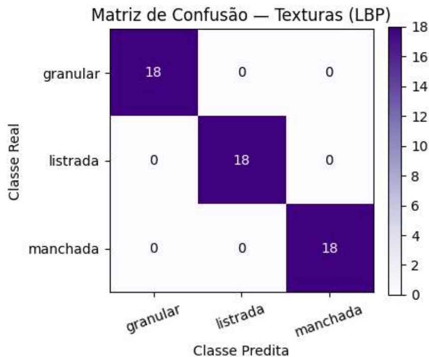
Figura 7.13: Matriz de confusão do classificador k-NN treinado com descritores LBP para as três classes de textura sintética.
