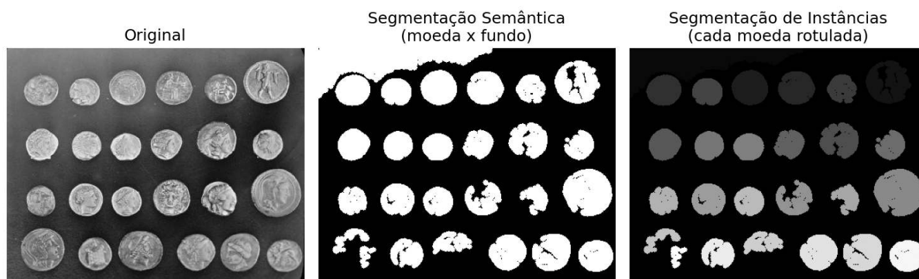
Figura 8.7: Segmentação clássica (não baseada em aprendizado profundo): máscara semântica (moeda x fundo) via limiarização de Otsu, e segmentação de instâncias via rotulagem de componentes conectados.
