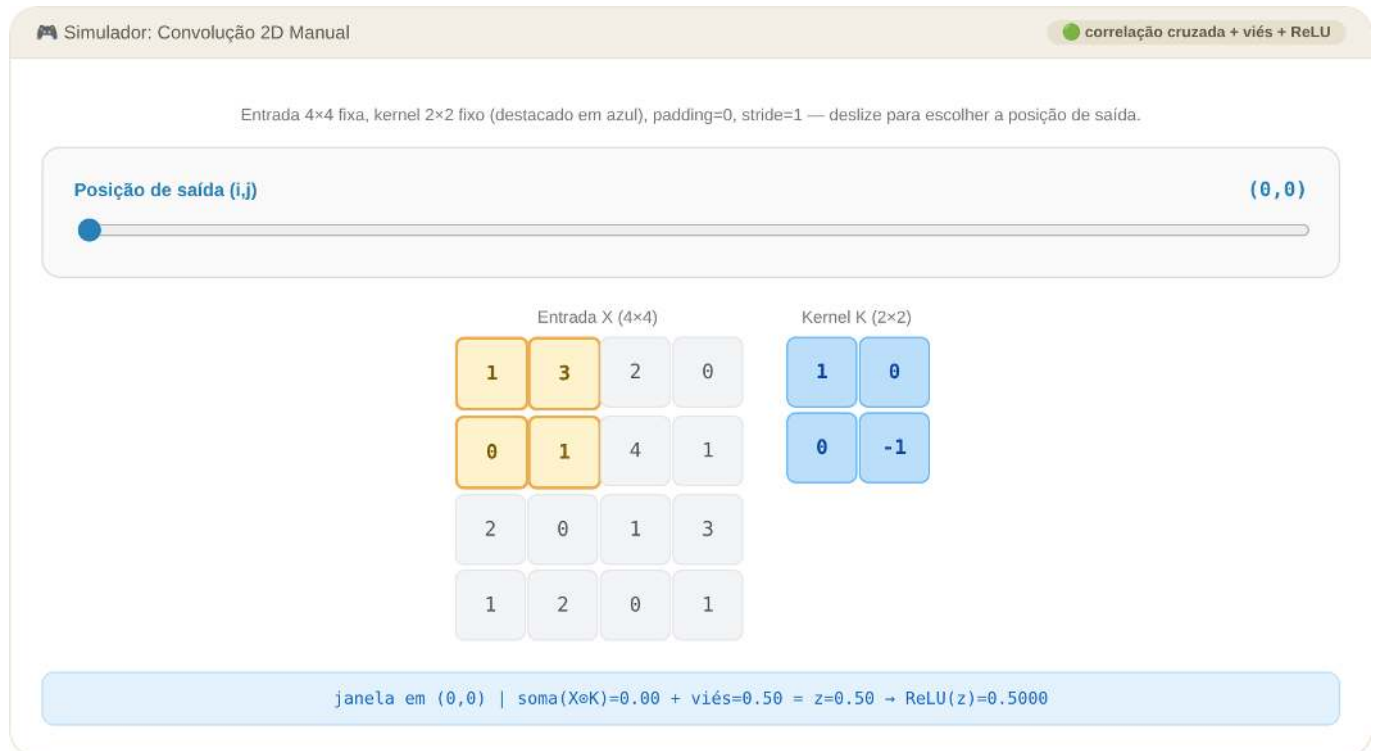
Figura 9.24: Simulador: Convolução 2D Manual (correlação cruzada + viés + ReLU)
