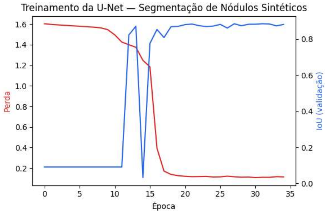
Figura 9.19: Curva de treinamento da U-Net compacta: perda de treinamento (entropia cruzada binária combinada à perda Dice) e IoU médio no conjunto de validação ao longo das épocas.
