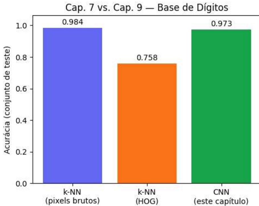
Figura 9.13: Comparação de acurácia entre os classificadores clássicos do Capítulo 7 (pixels brutos e HOG com k-NN) e a CNN treinada neste capítulo, na mesma base de dígitos.
