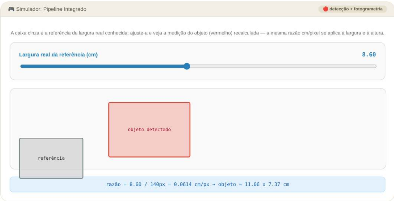
Figura 9.28: Simulador: Pipeline Integrado — NMS + Medição por Referência de Escala
