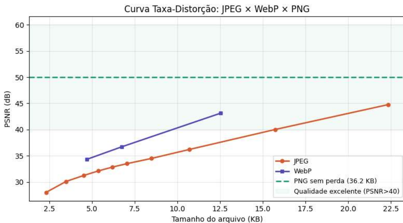
Figura 5.27: Curva taxa-distorção: PSNR vs tamanho de arquivo para JPEG, WebP e PNG aplicada à imagem do Cameraman .
