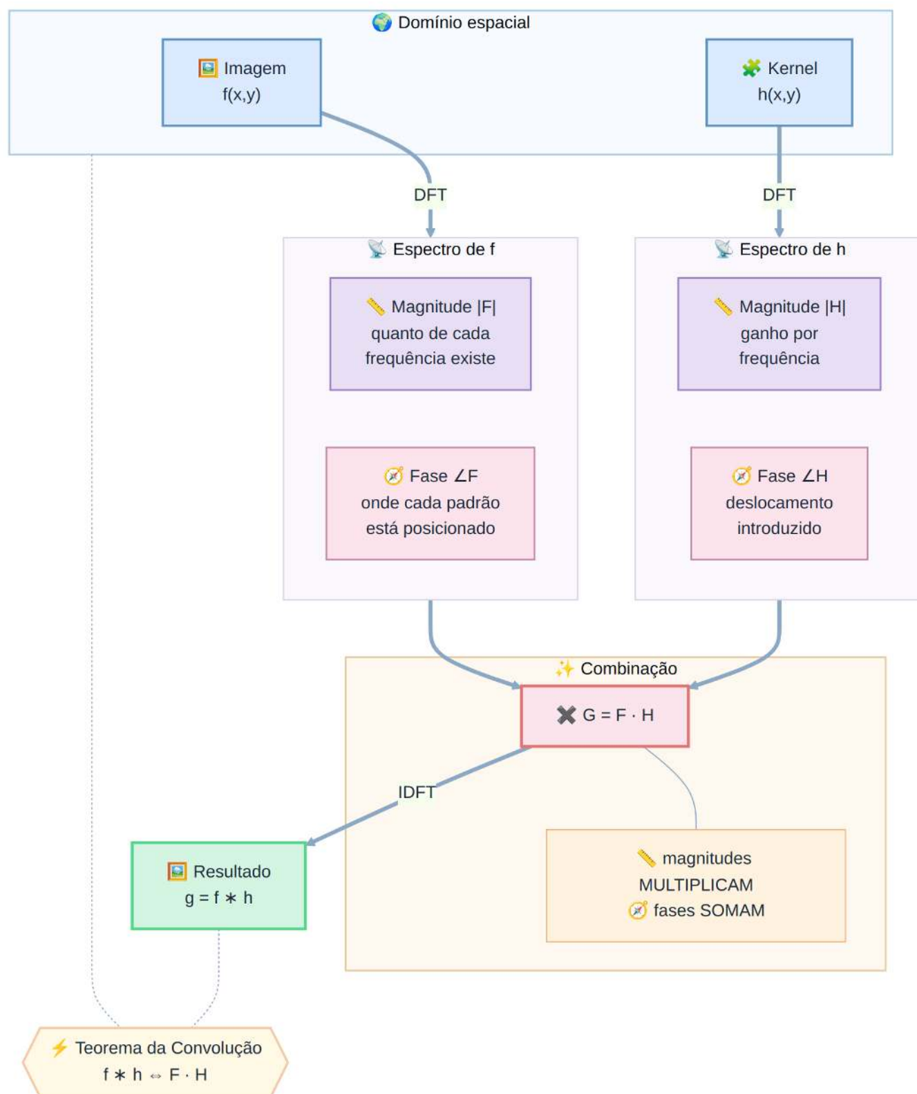
Figura 5.30: Mapa conceitual das transformações e propriedades no domínio da frequência.
